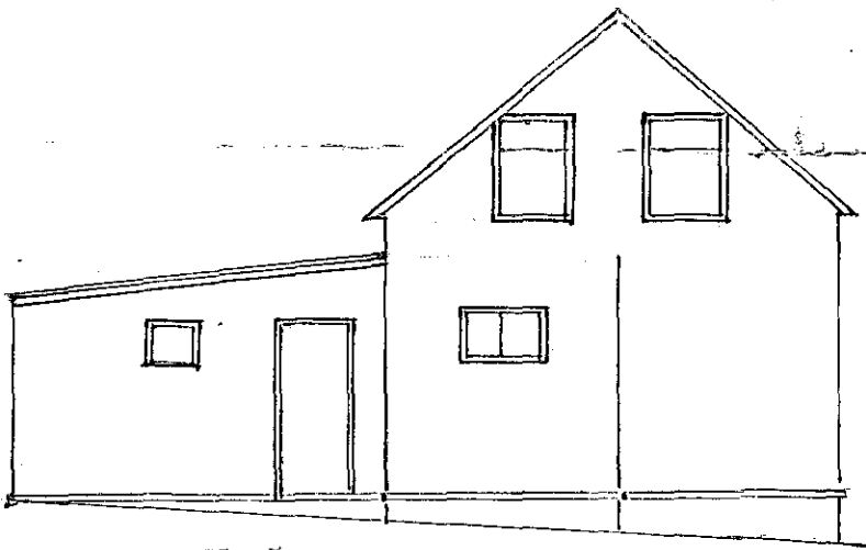
Norðurgafll.
