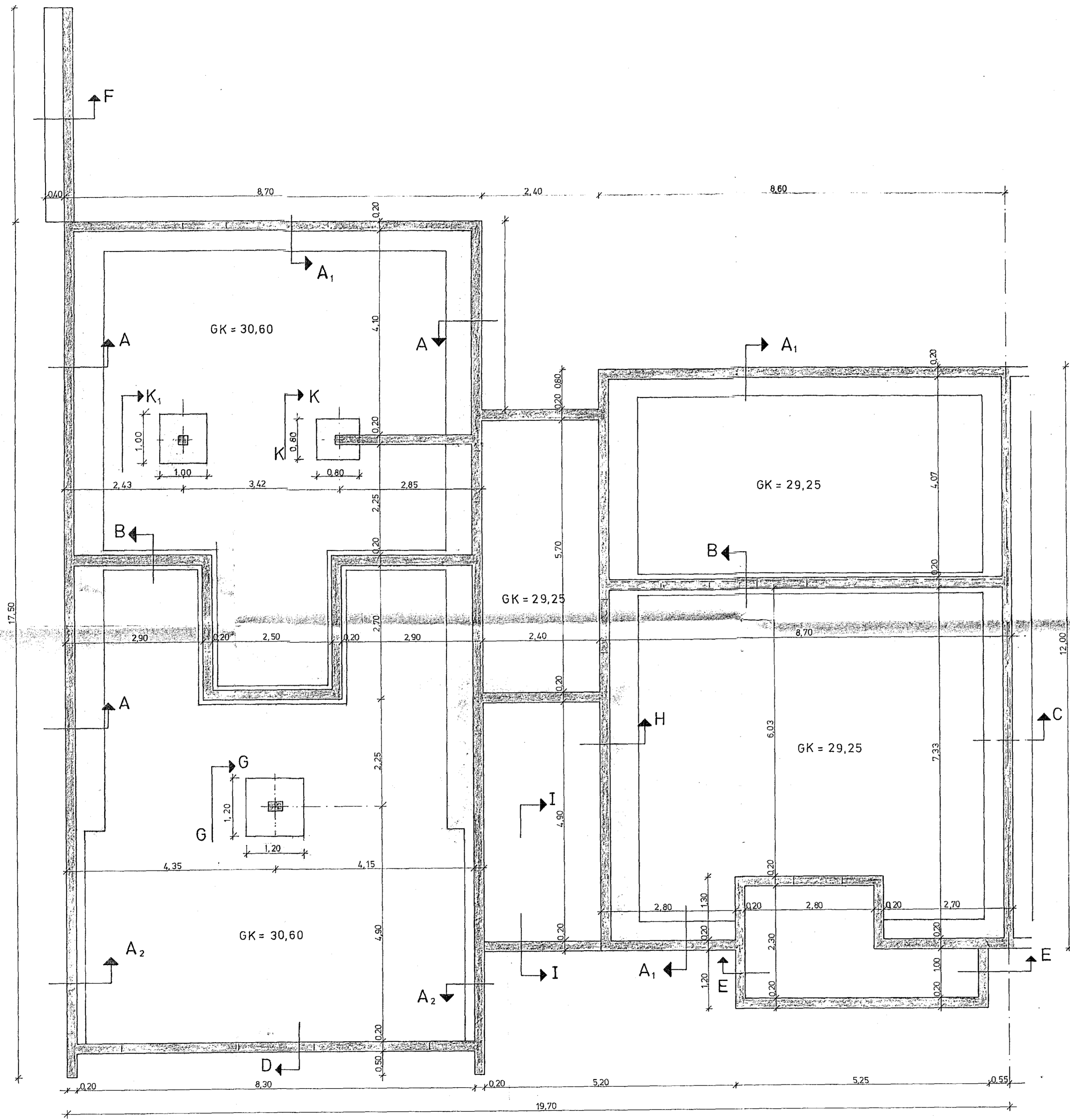
GRUNNMYND 1 : 50
