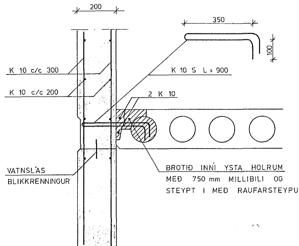
SNID 'I HLIÐARVEGG 1:10
