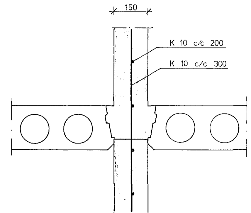
SNID 'I MILLIVEGG 1:10
