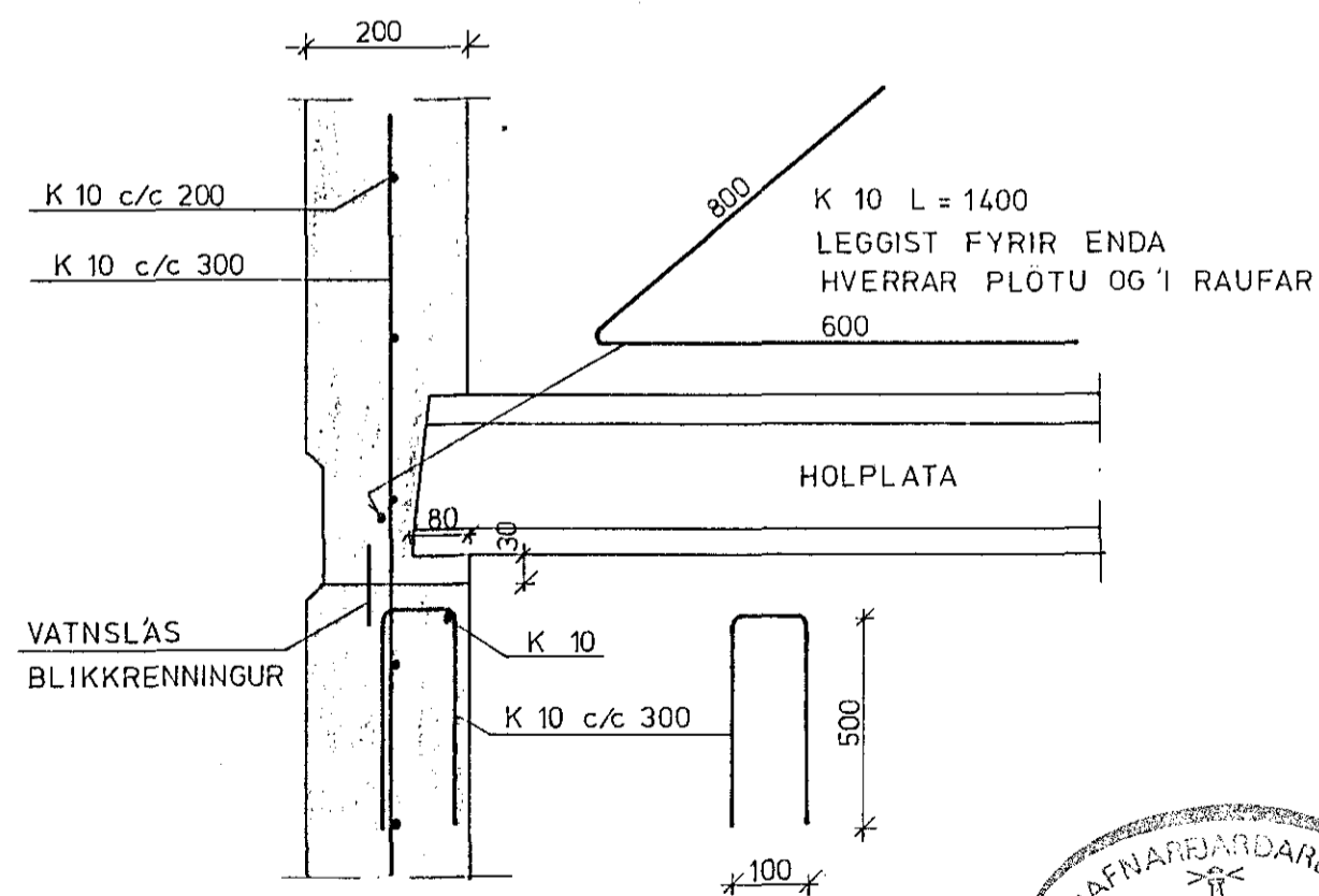
SNID 'I STAFNVEGG 1:10
