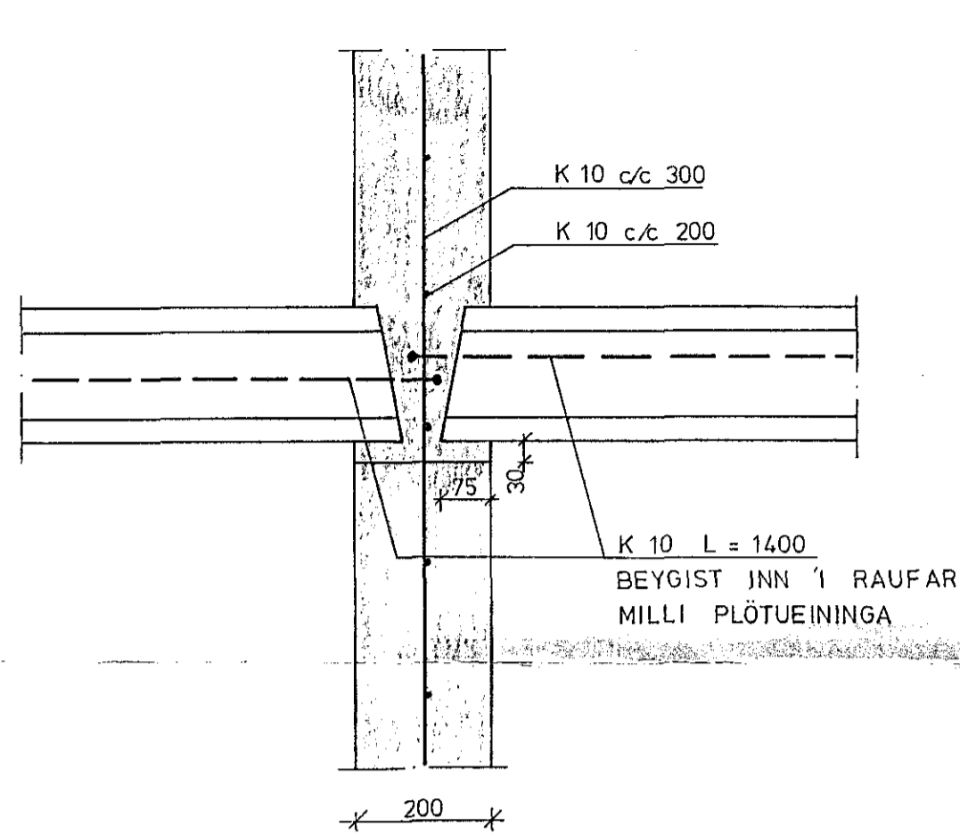
SNID 'I VEGG MILLI HÚSA NR. 11 OG 13
