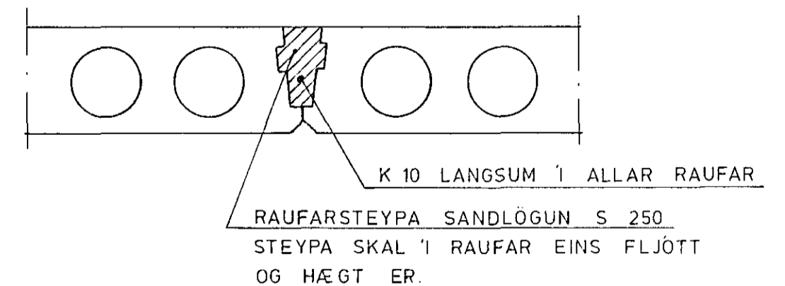
SNID 'I RAUF 1:10
