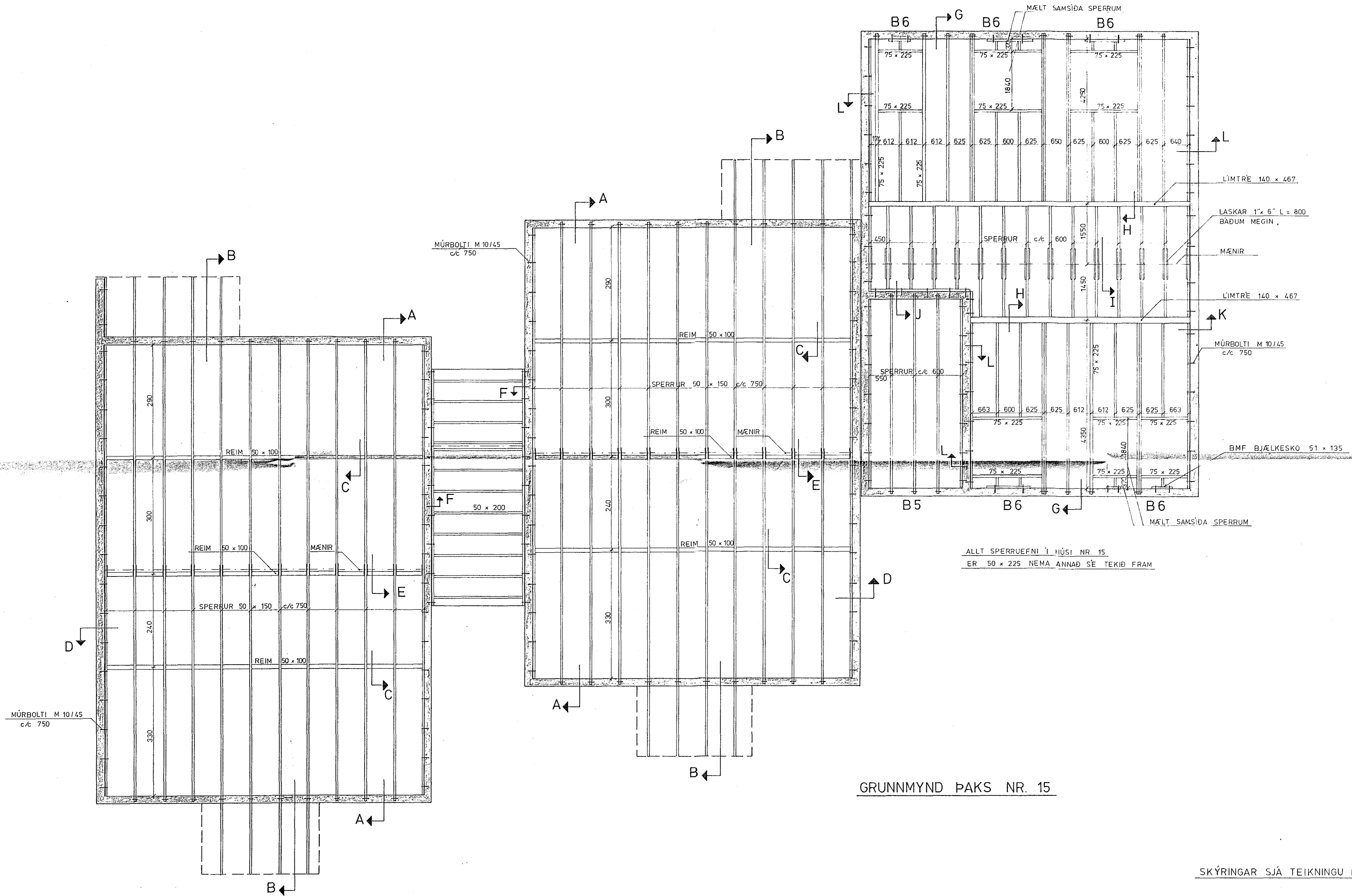
GRUNNMYND PAKS NR. 13
