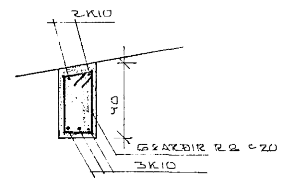
SNID Í BITA Y BILG. 1:20
