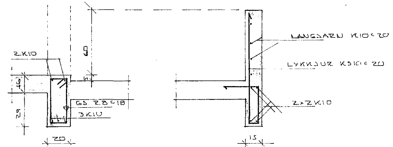
SNID Í GLUGGA OG SVALAHANDRÍÐ 1:20
