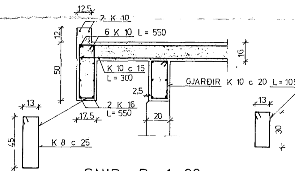
SNID D 1:20
