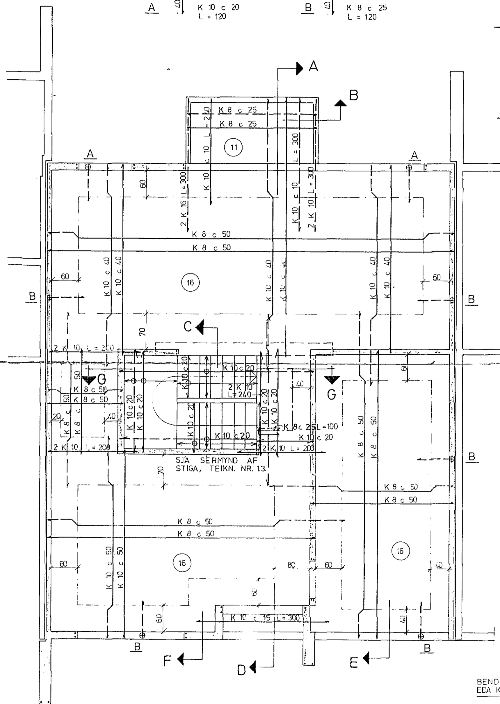
GRUNNMYND 1:50
