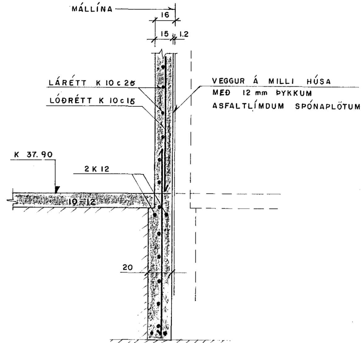
SNID C Mkv. 1:20
