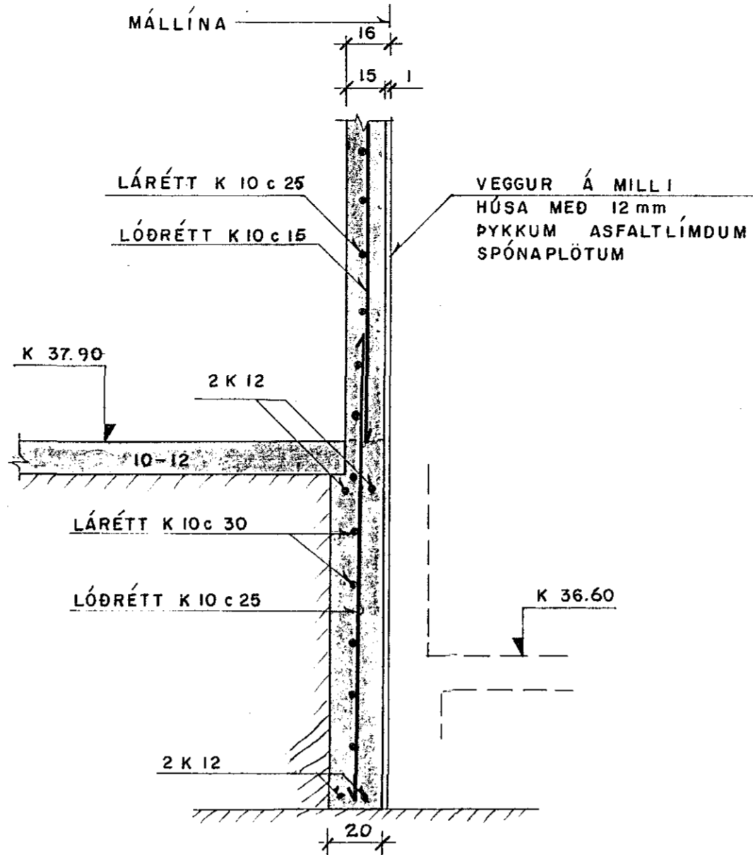
SNID B Mkv. 1:20
