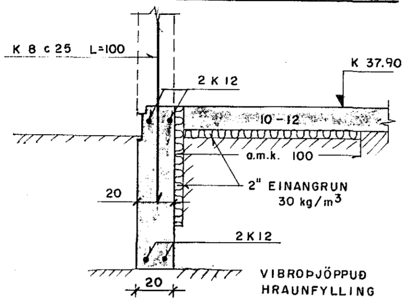
SNID A Mkv. 1:20
