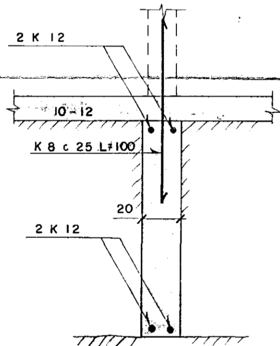
SNID D Mkv. 1:20
