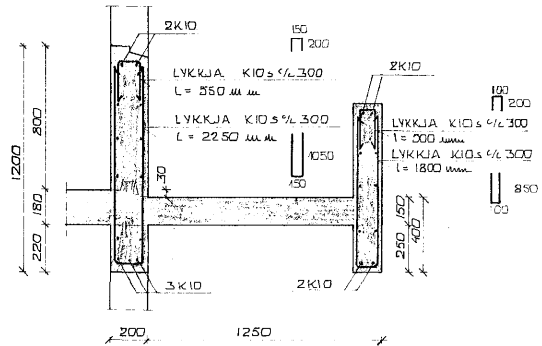
SNID A-A. Mkv. 1:20
