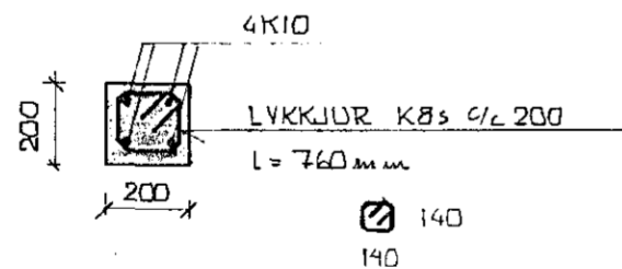
SULA S1.1. Mkv. 1:20
