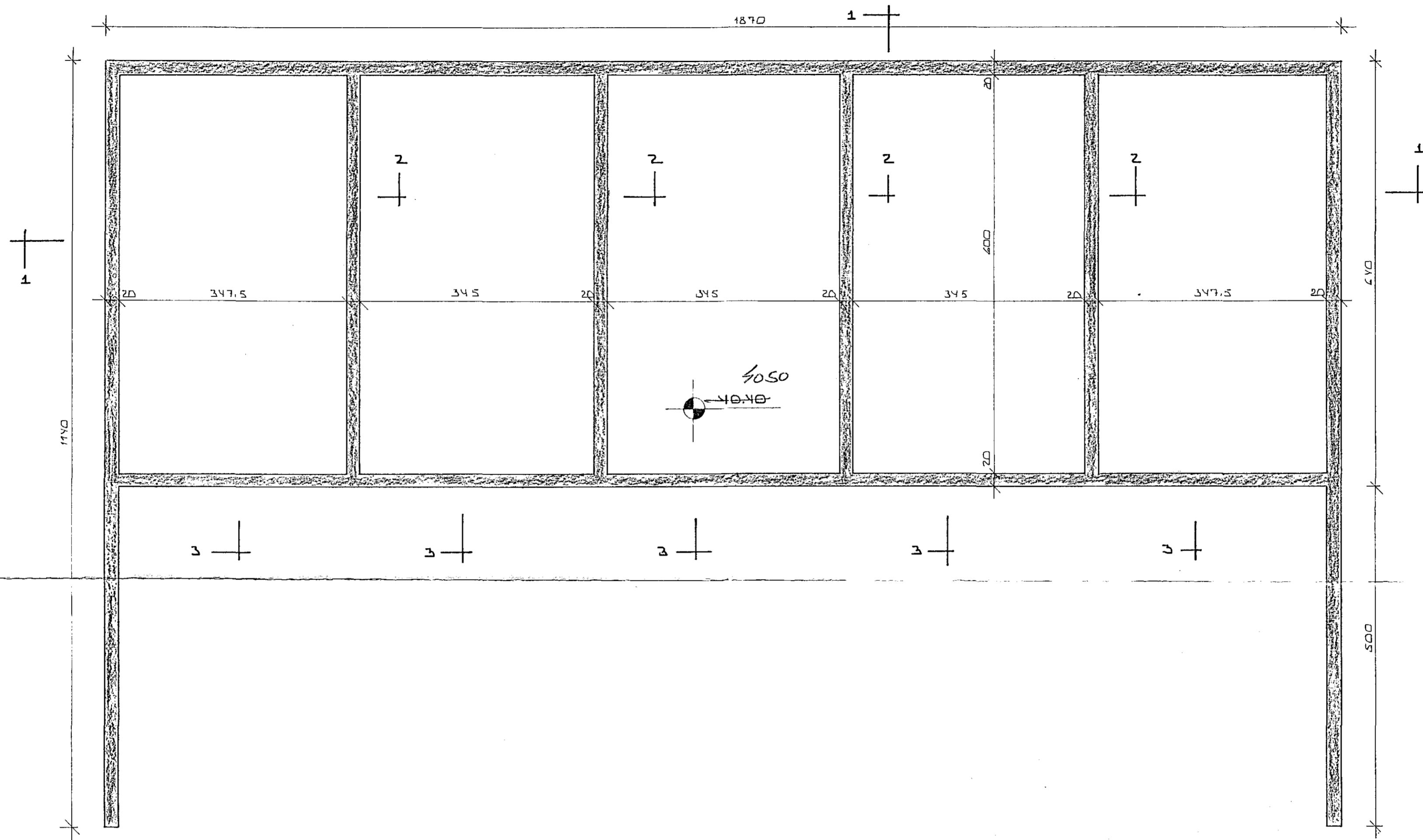
GRUNNMYND ~ 1:50
