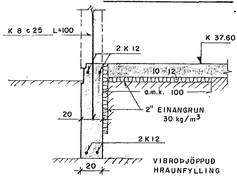
SNID A Mkv. 1:20
