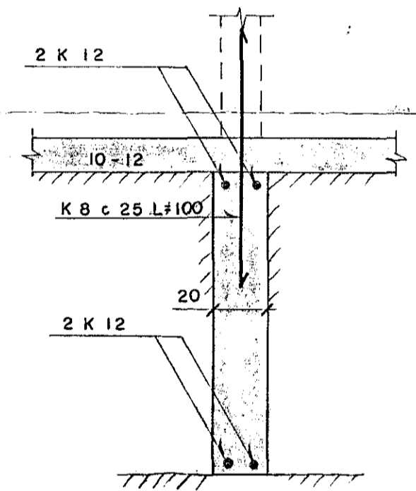
SNID D Mkv. 1:20
