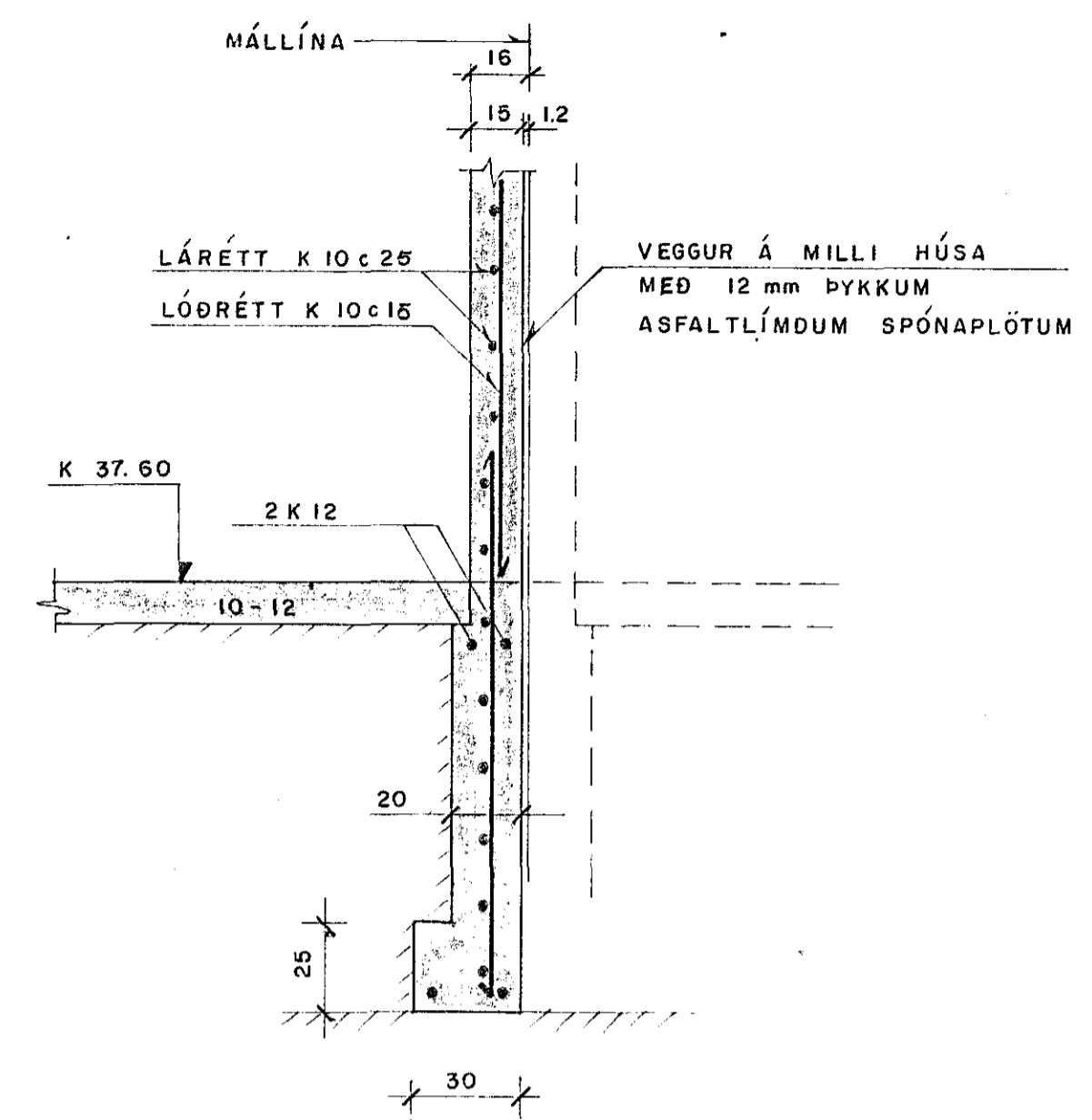
SNID C Mkv. 1:20
