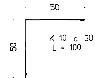
STÁLVINKILL A
