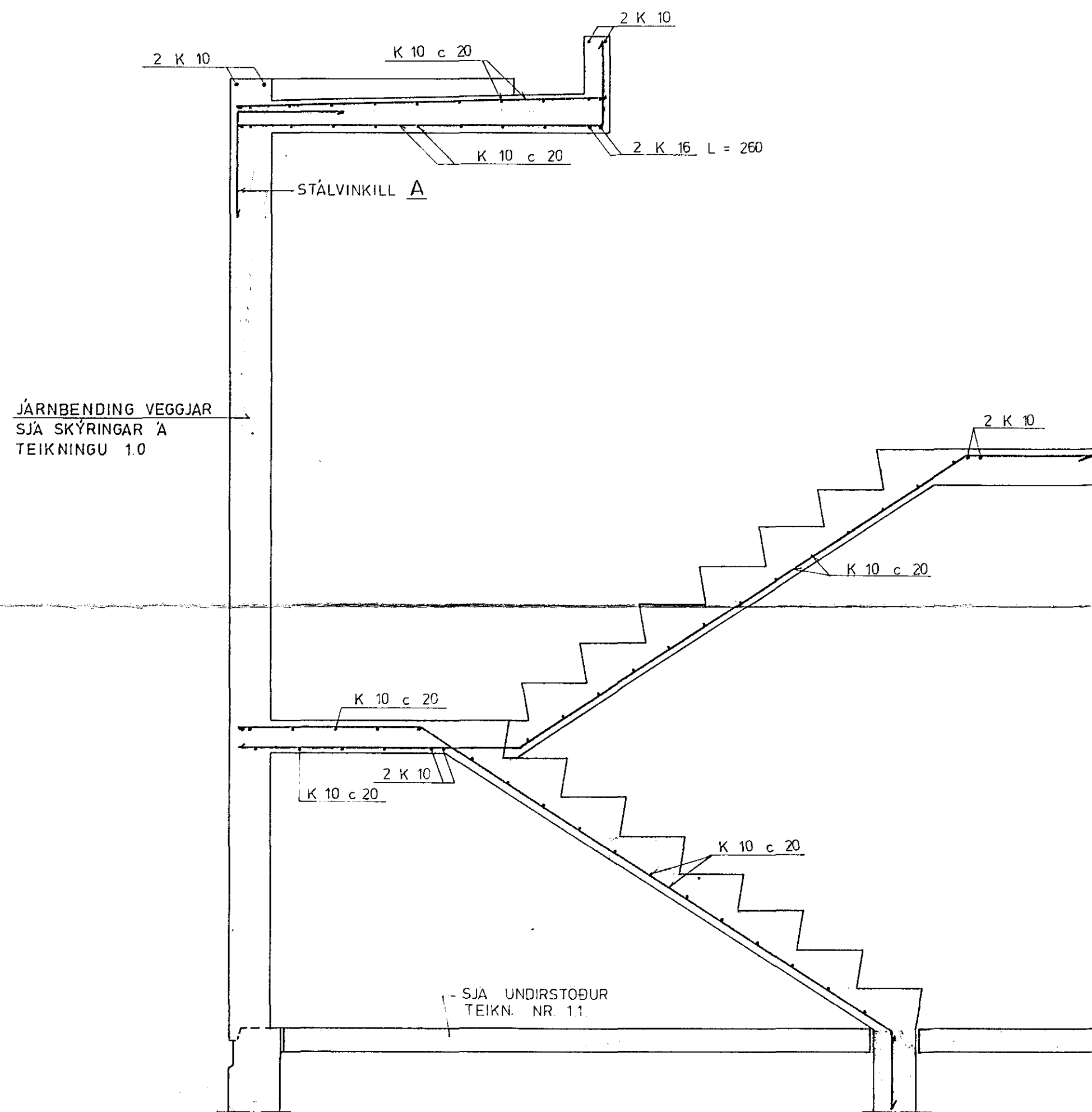
SNID '1 STIGAHÚS 1:20
