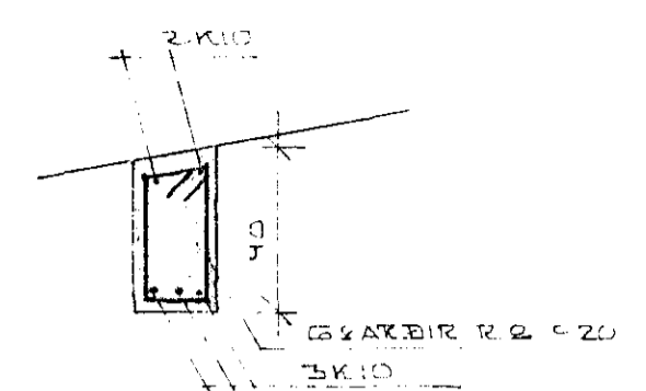
SNID Í BITA Y BILG. 1:20
