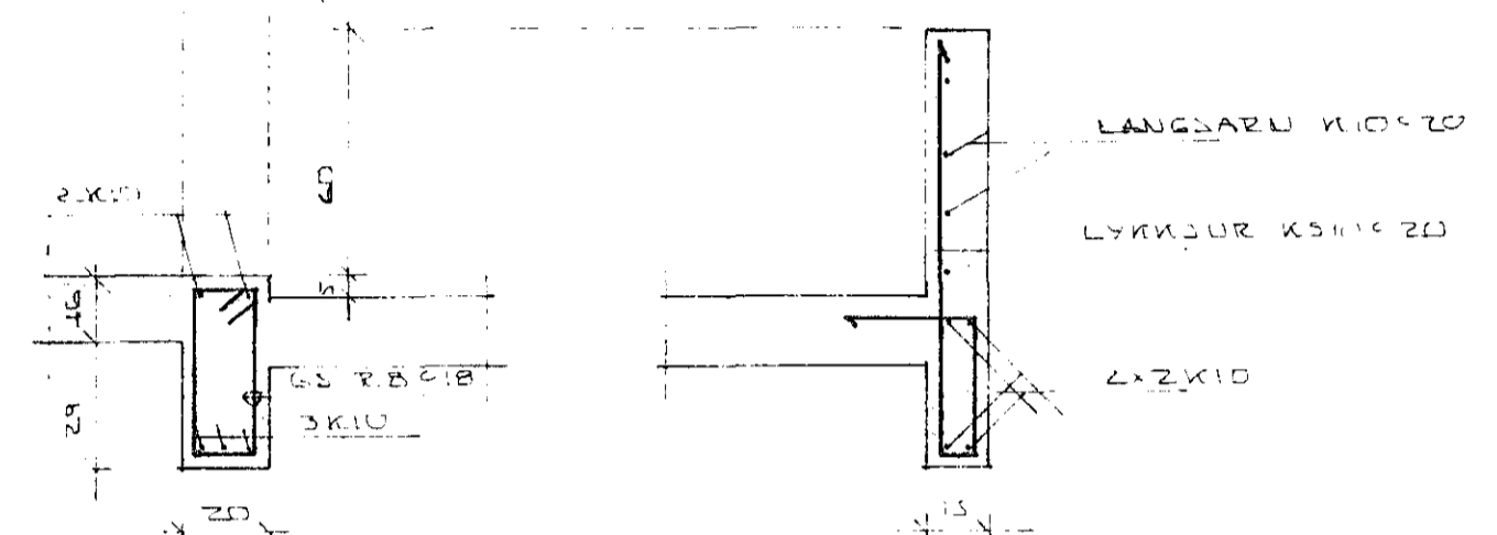
SNID Í GLUGGA OG SVALAHANDRÍÐ 1:20
