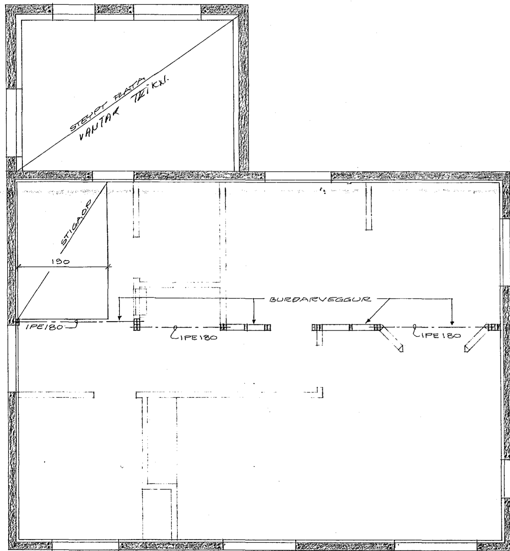
BURDARVEGGUR OG STÁLBITAR UNDIR GÖLF GRUNNMÝND, M=1:850
