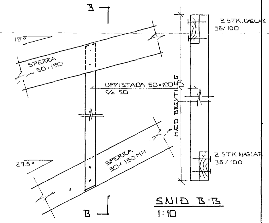
SÆRMYND I KVISTVEGGI VIÐ ÞAK 1:10
