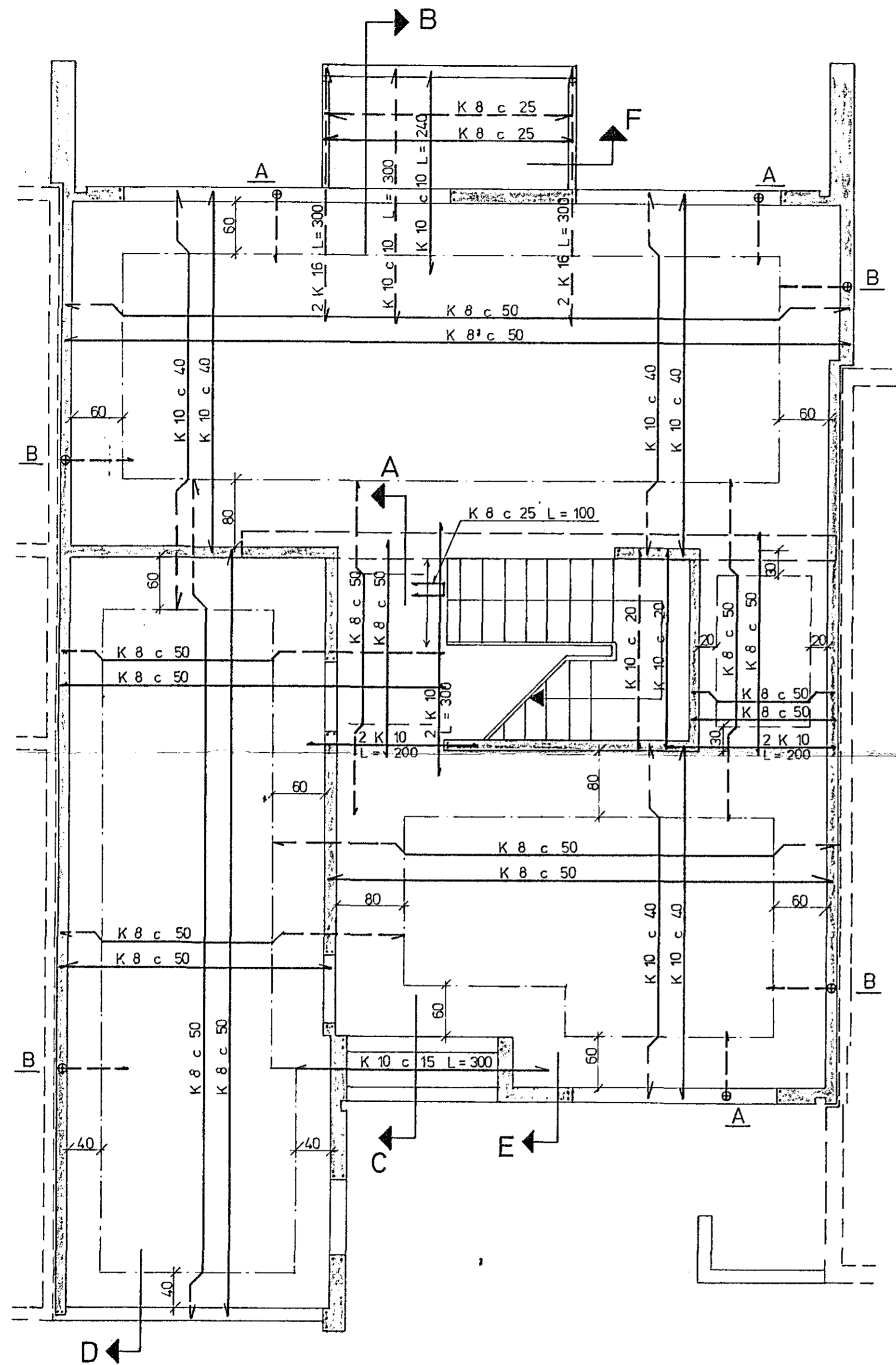
GRUNNMYND 1 : 50
