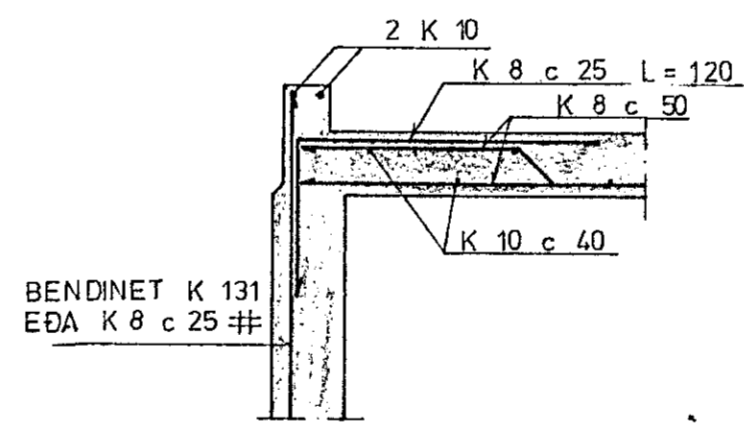
SNID E 1 : 20
