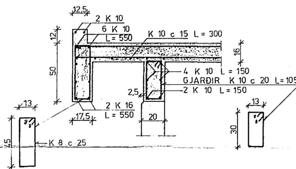
SNID C 1 : 20
