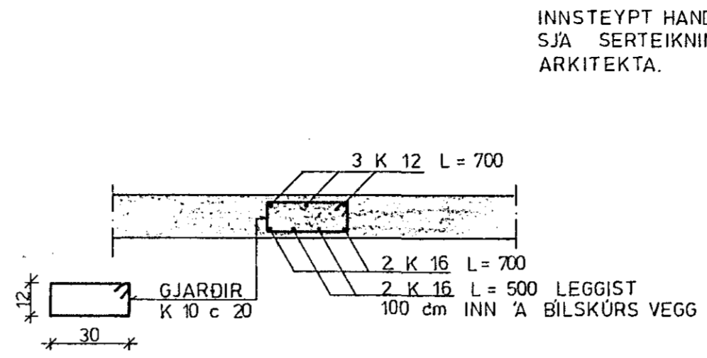
SNID A 1 : 20
