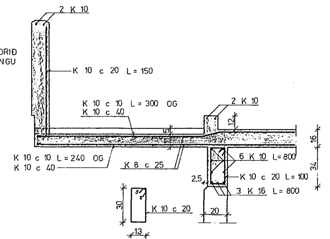
SNID B 1 : 20
