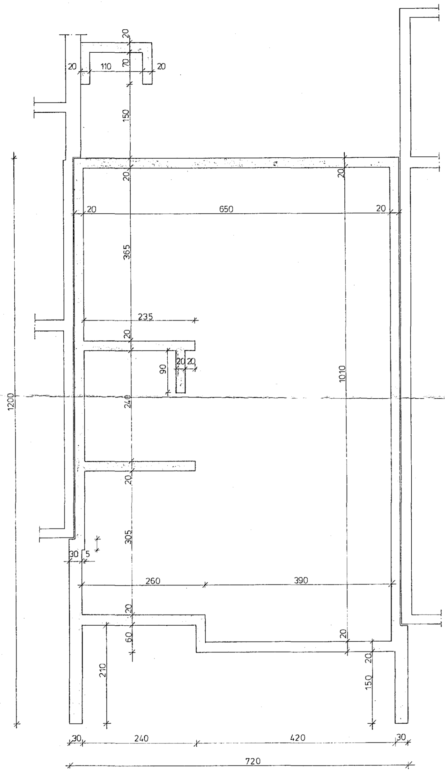
GRUNNMYND 1:50
