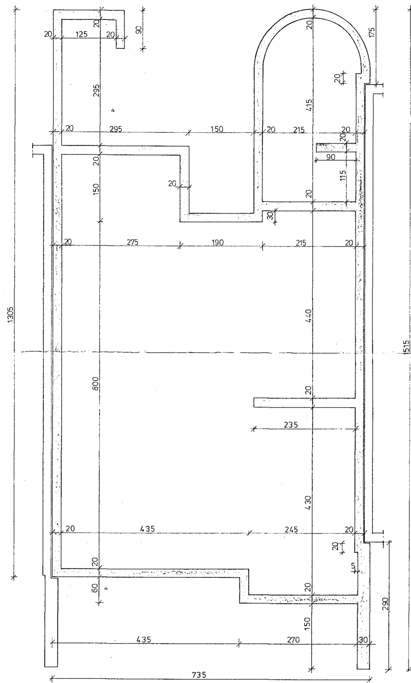
GRUNNMYND 1:50
