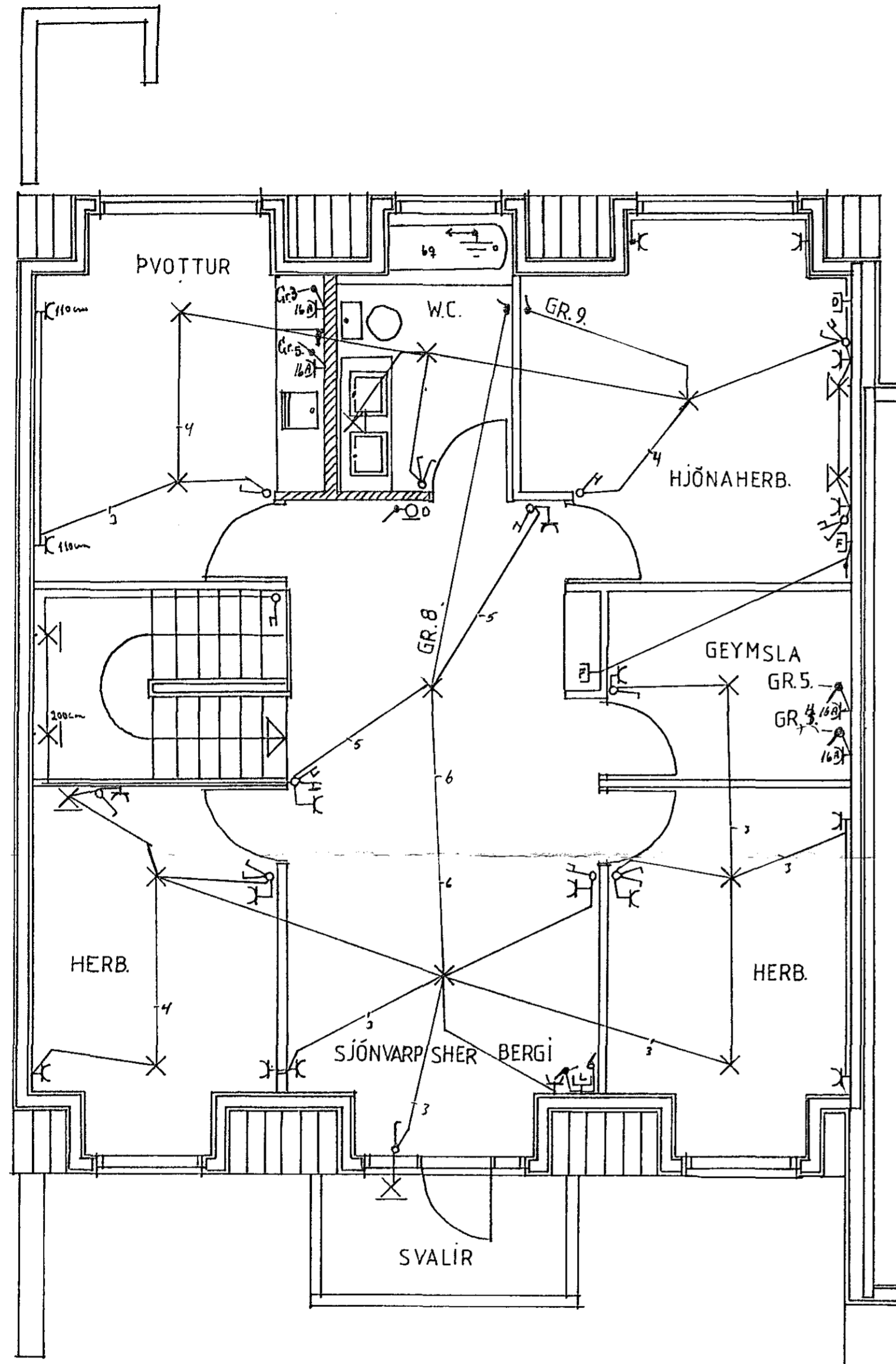
2 HÆÐ GRUNNMYND. 1:50
