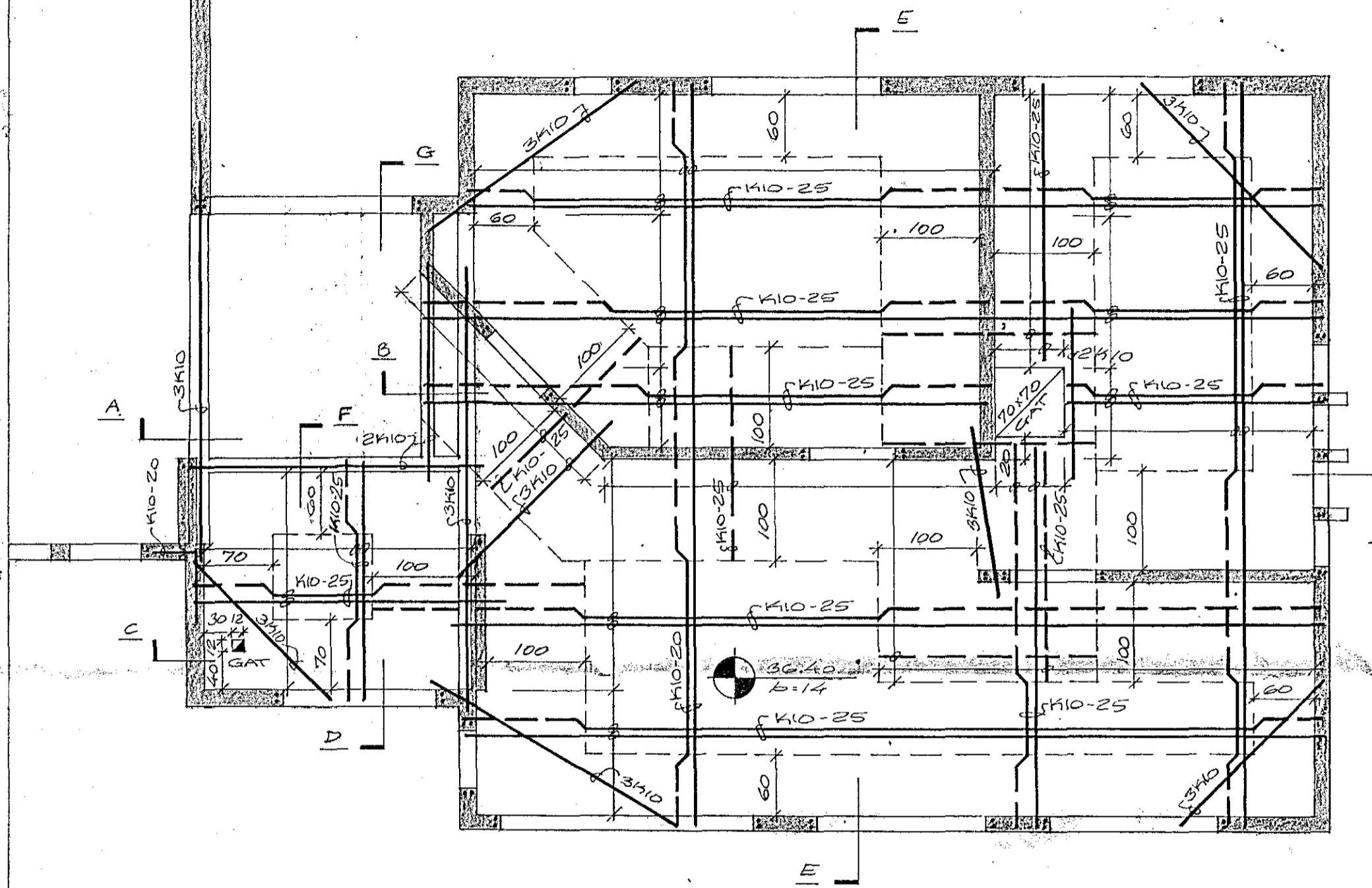
GRUNDMYND, M=1:350
