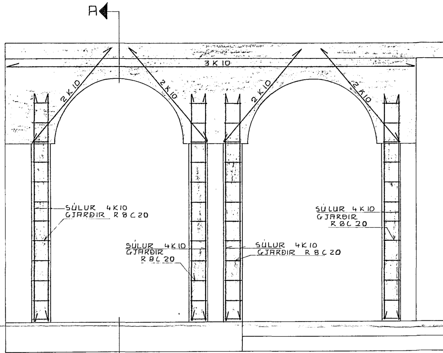
SÚLUR OG BITI INNI 1:20
