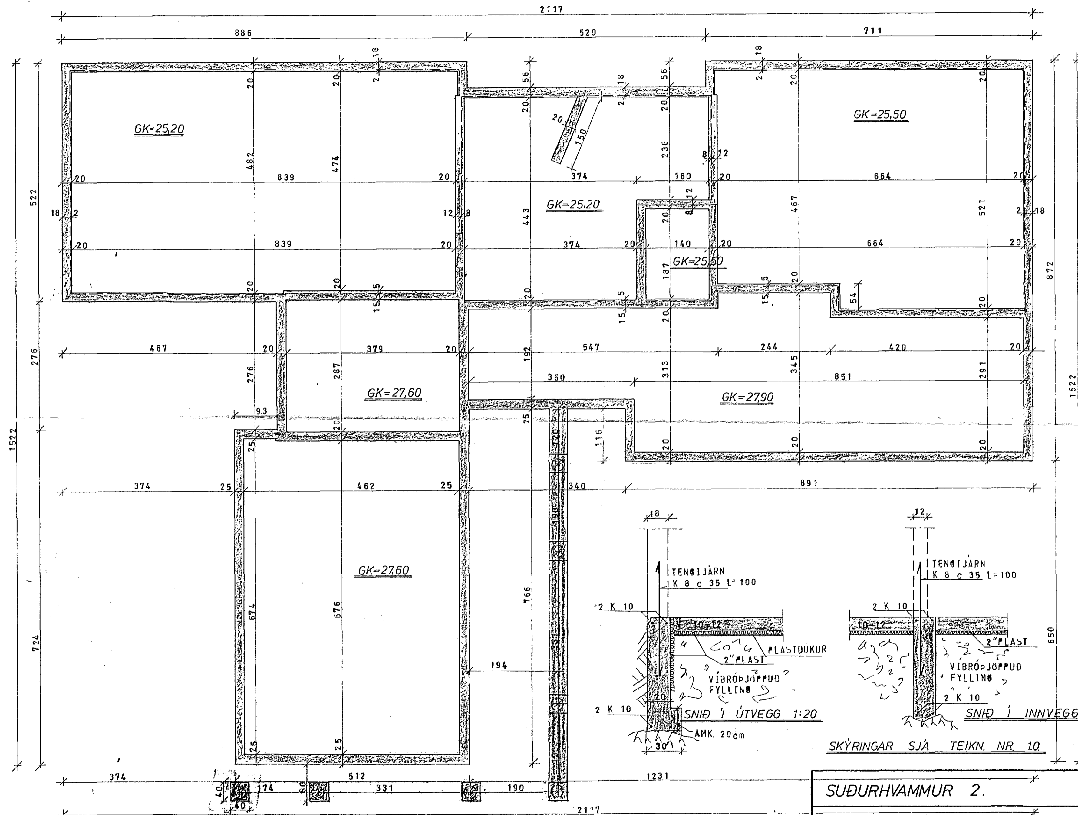
GRUNNMYND — UNDIRSTÖÐUR 1:50
