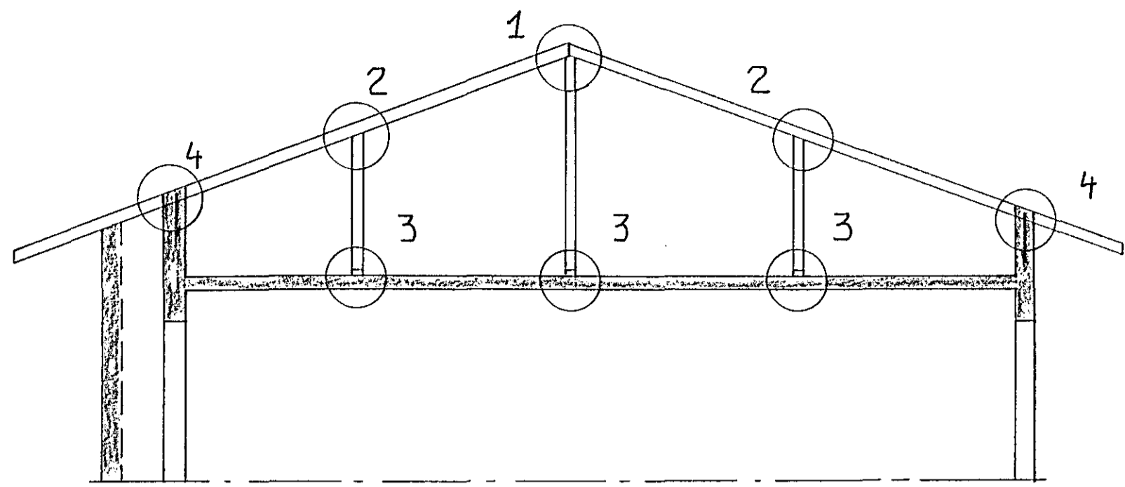
SNID A-A 1:50
