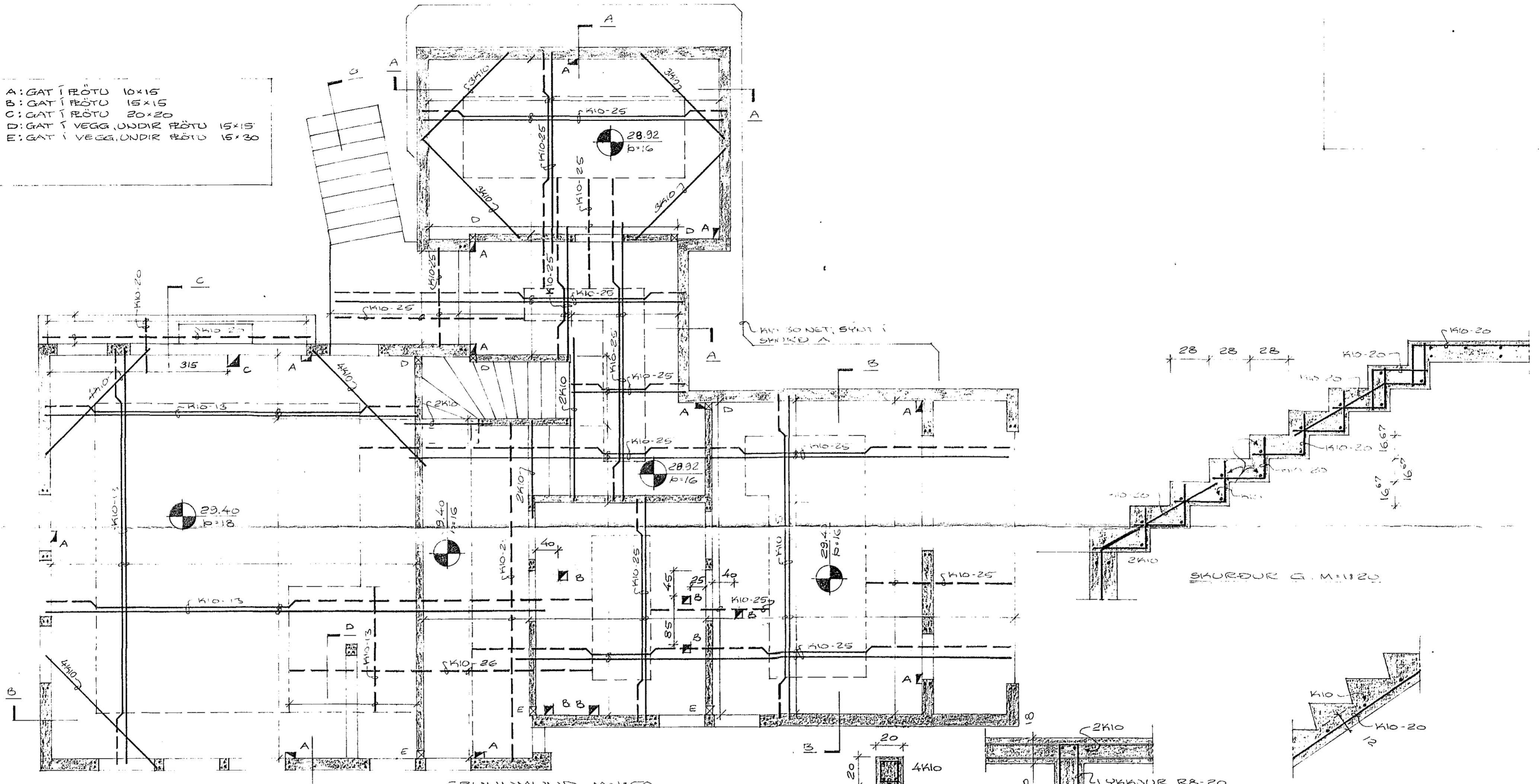
GRUNNMYND, M=1:50
