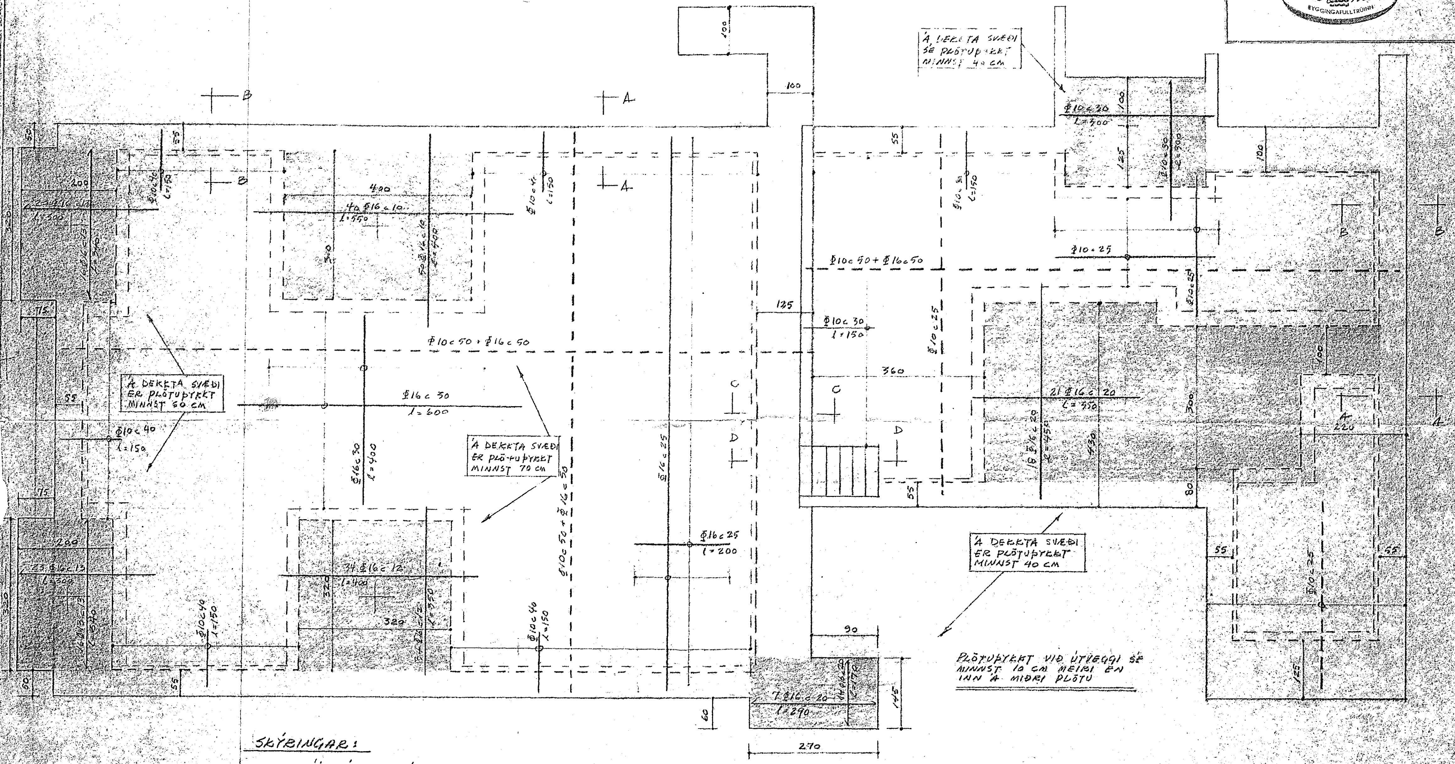
GRUNNPLATA OG SÖKKLAR 1:50
