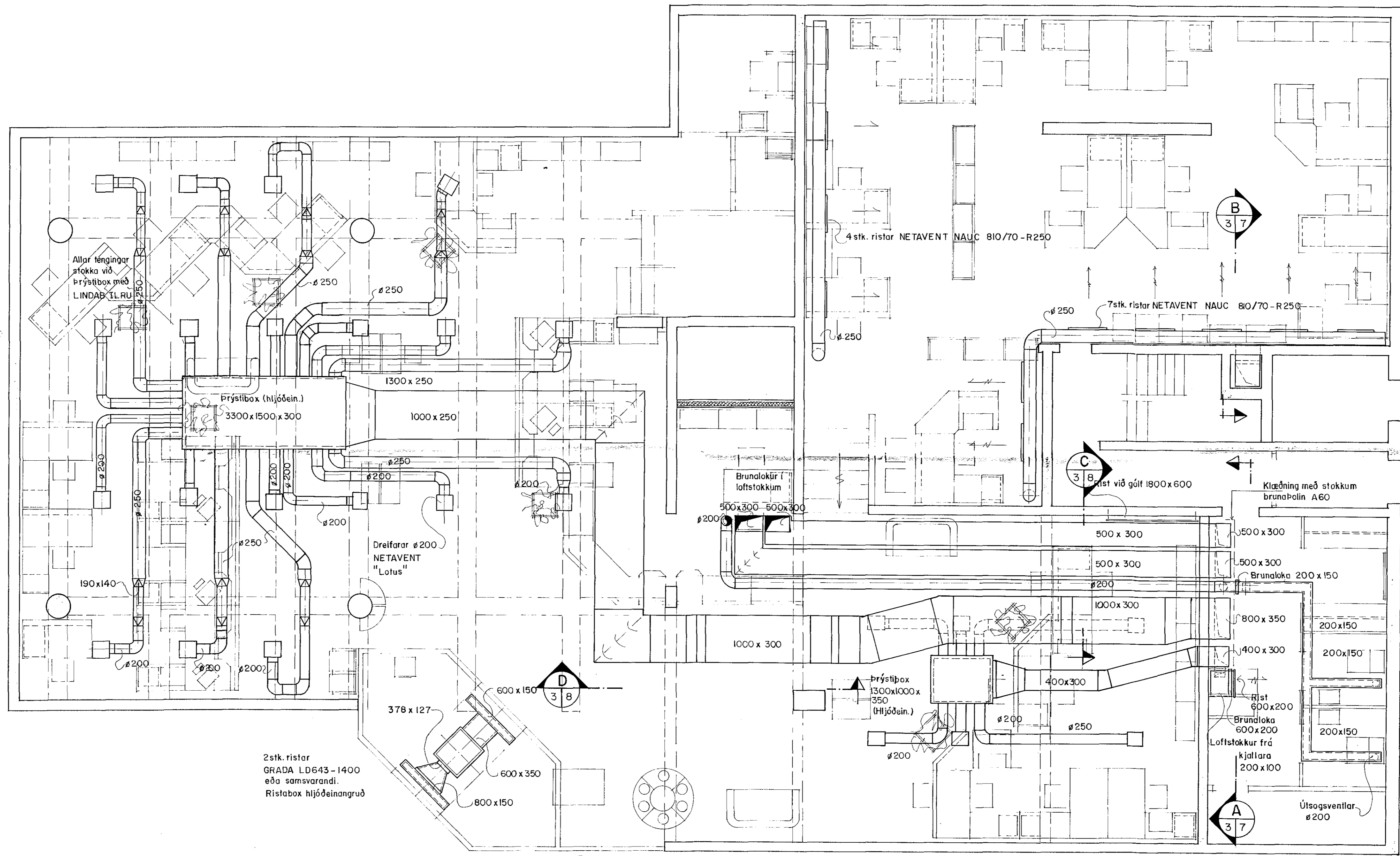
Anddyrissamstæða 800 m 3 /l
