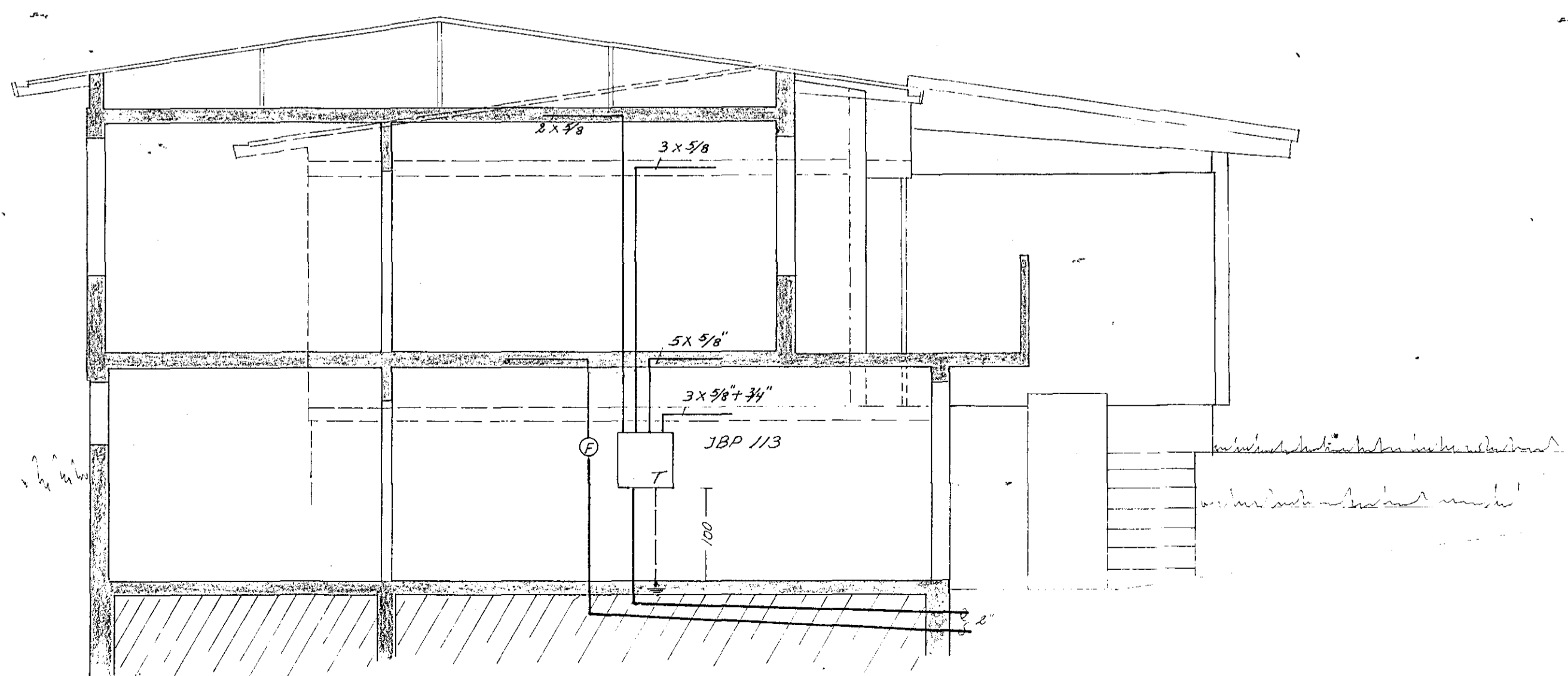
snid A-A
