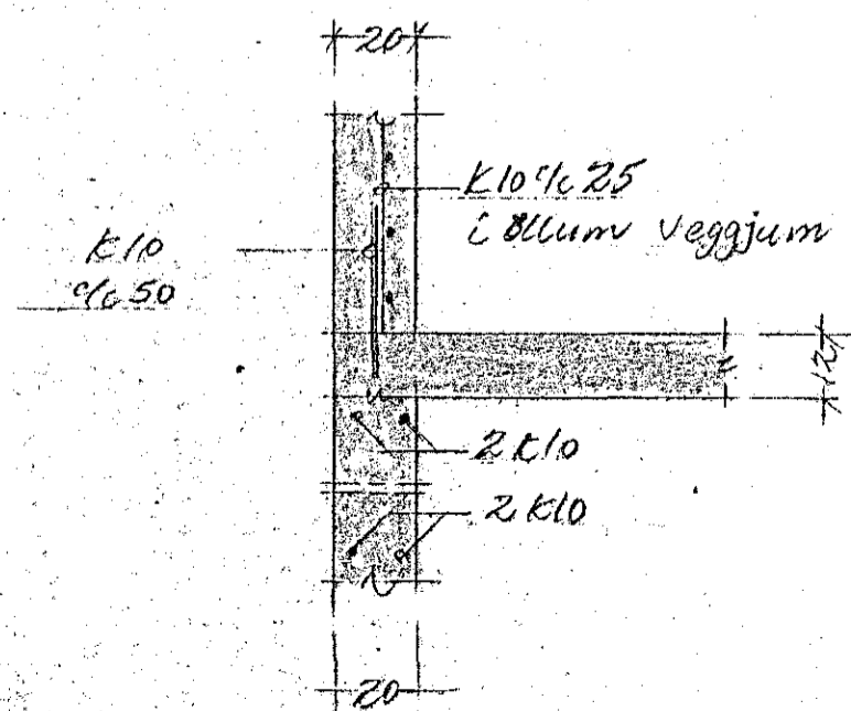
Snit A-A
