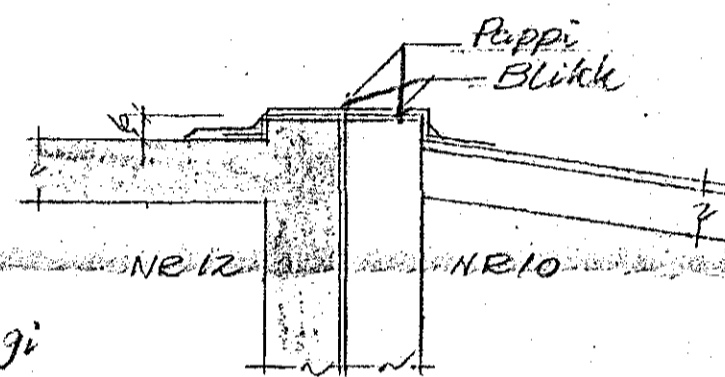
Snit C-C
