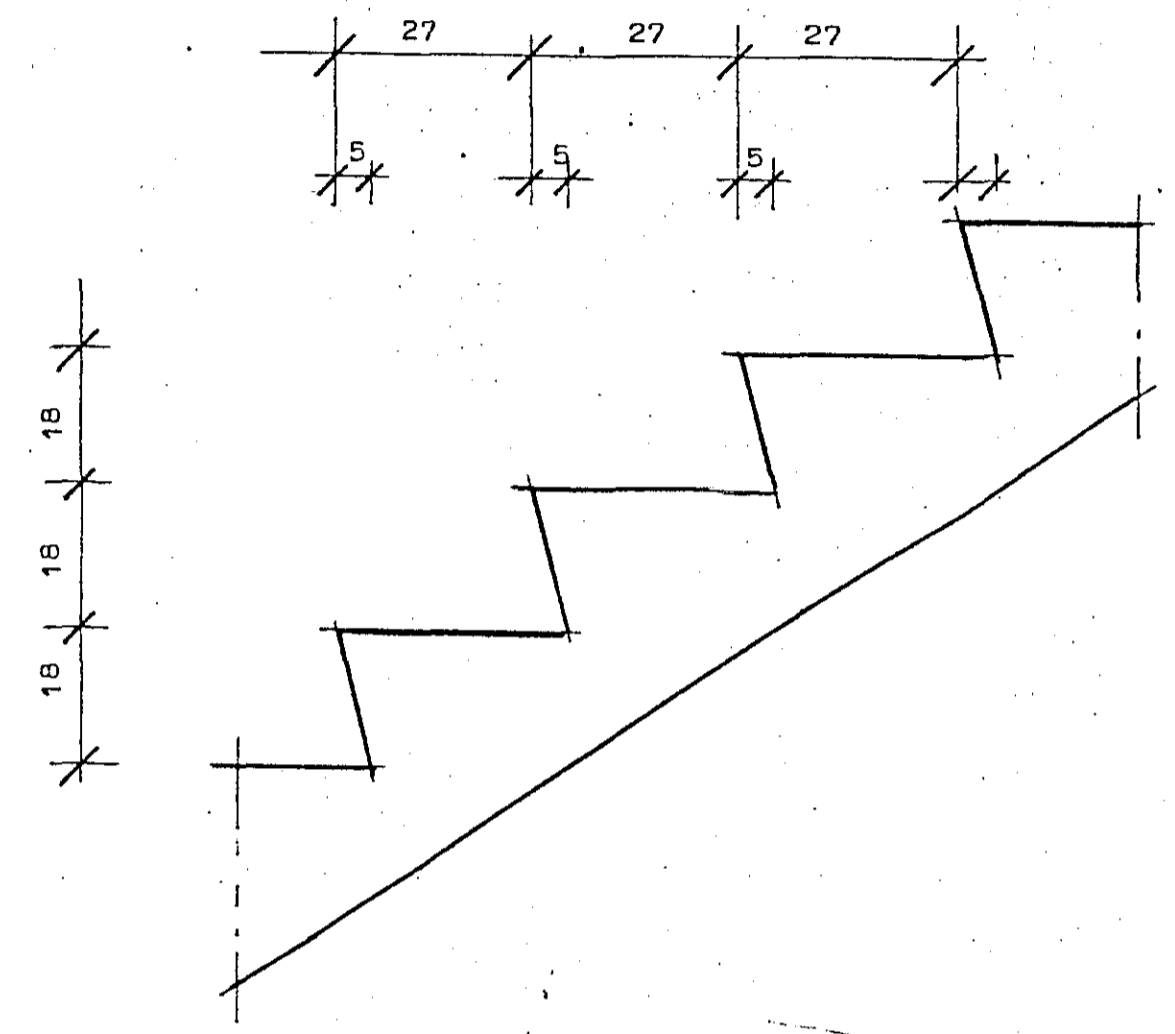
Sneiðing í stiga í ganglinu Mk 1:10
