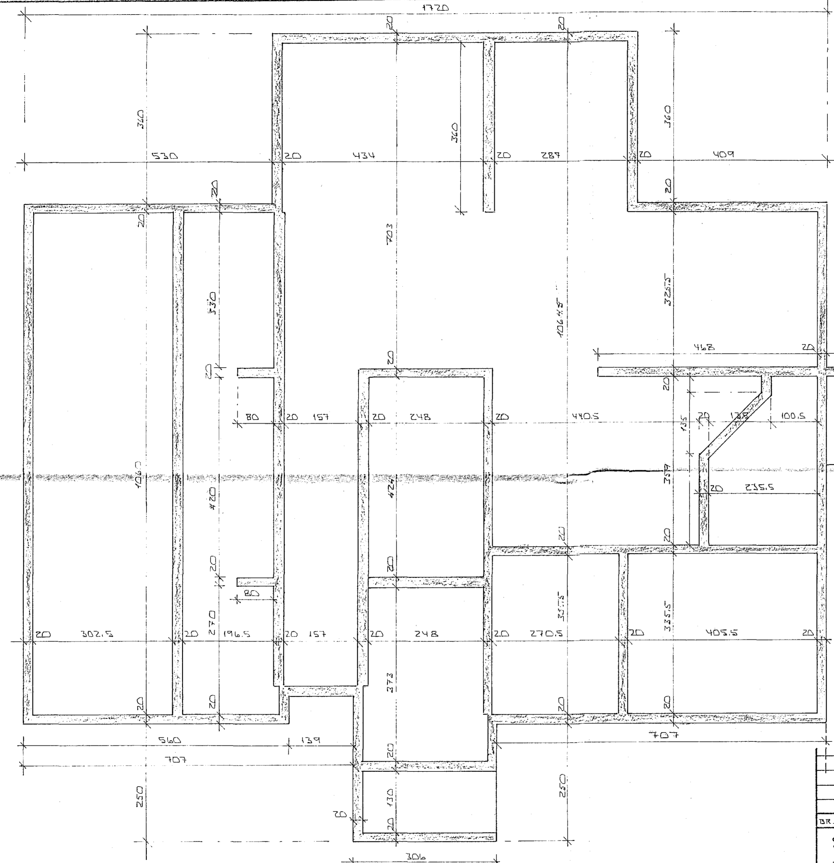
GRUNNMYND UNDIRSTÖÐUR 1:50
