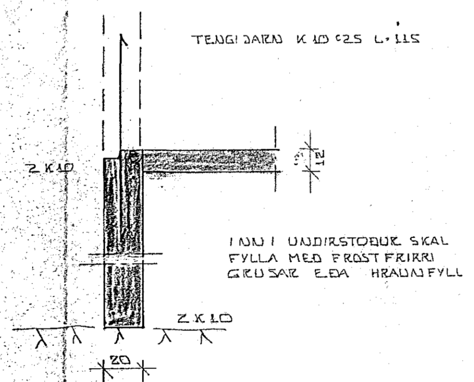
SNID I ÚTV. 1:20
