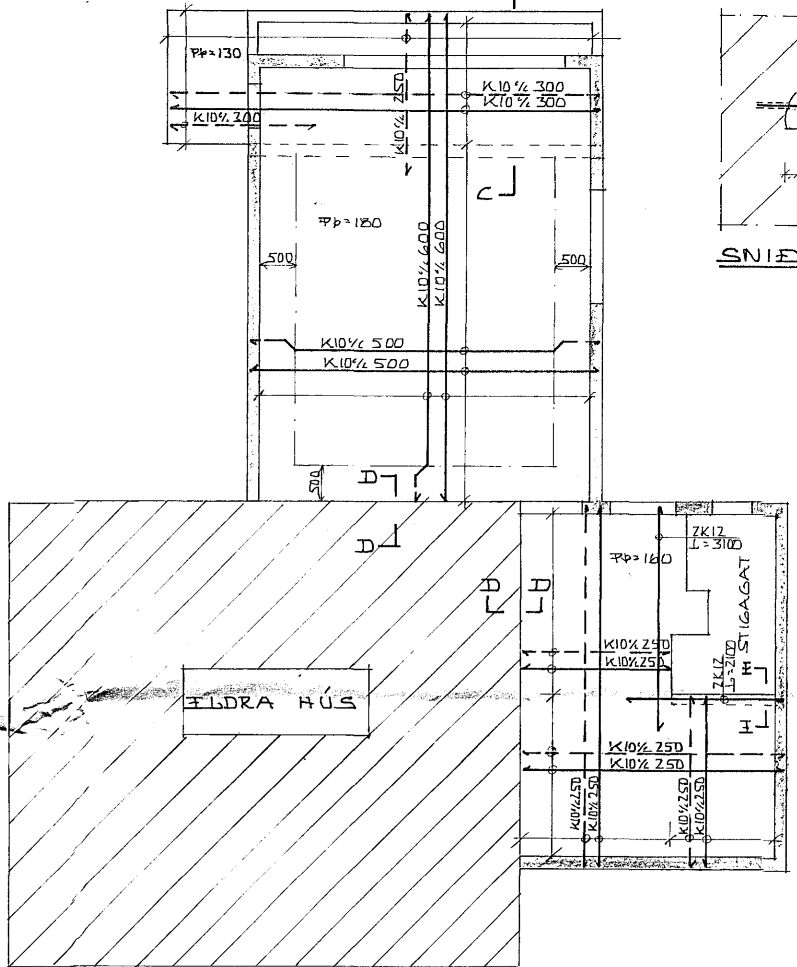
JÄRNBINDING LOFTPLÖTU GRUNNMYND 1:50
