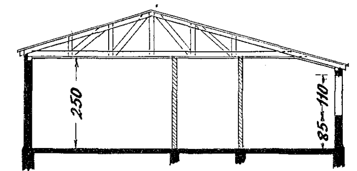
Þverskurður
