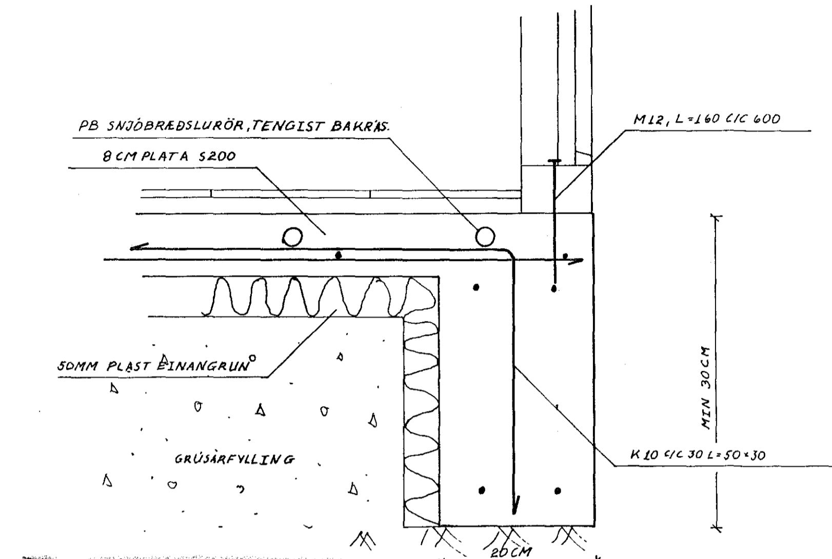
SNID A-A, M 1:5
