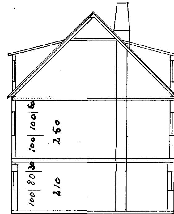
Skurður
