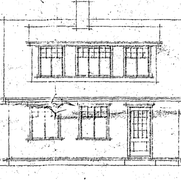
AUSTURVEGGUR
