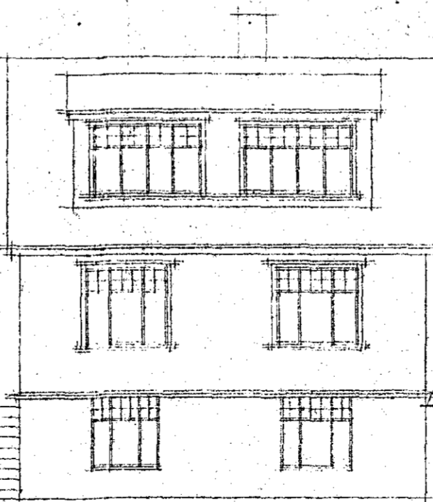
NORÐURVEGGUR
