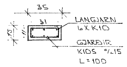
SÚLA S2 ~ 1:20
