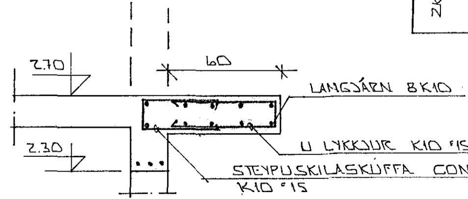
SNIED A Í SKYGGNI 1:20
