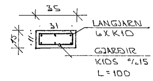
SÚLA S 1 ~ 1:20
