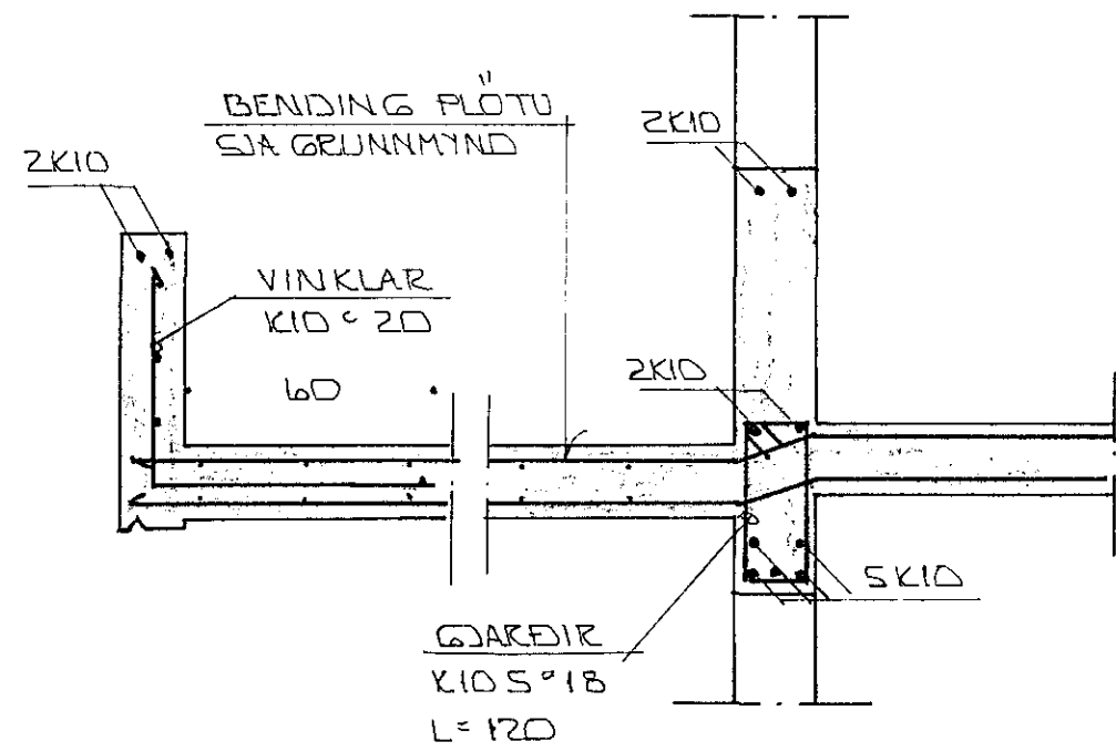
SNED 5 - 5 Í SVÁLIR 1:20
