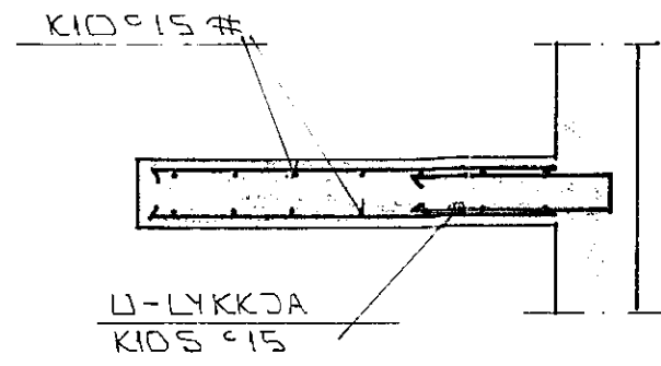
SNED 7 Í SKYGGNI 1:20
