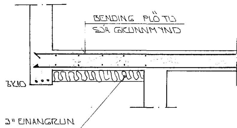
SNED 6 Í ÚTKRÖGUN YFIR KJALLARA 1:20
