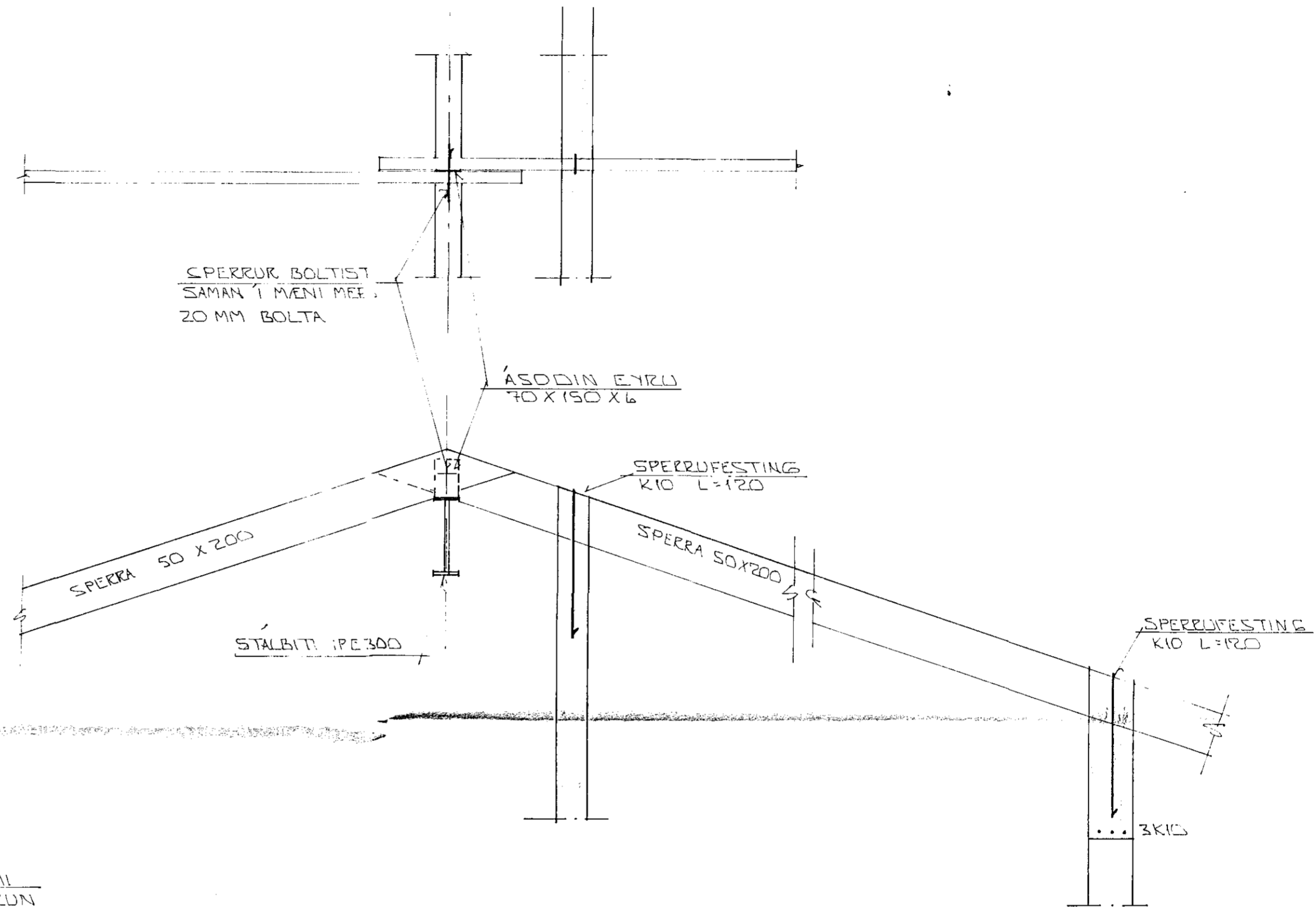
SNID 9 - 9 ~ 1:20 SJA BL. NR. 1-08
