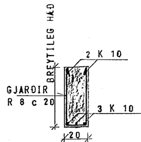
SNÍÐ A 1:20
