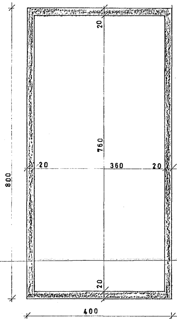
UNDIRSTÖÐUR 1:50
