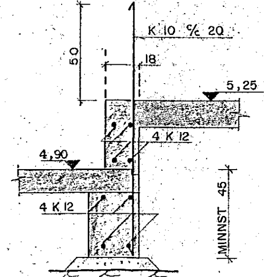
SNID V-V M. 1:20
