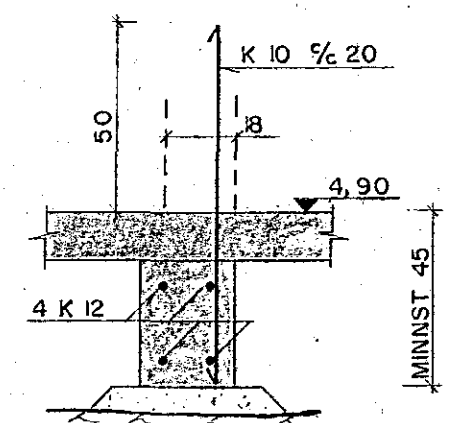
SNID U-U M. 1:20
