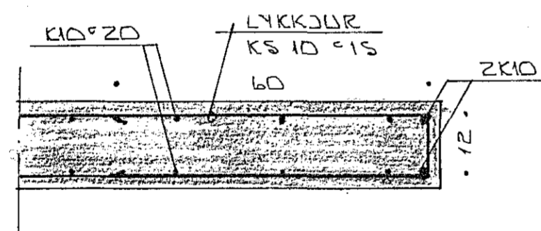
SNID 5 Í SVALIR • 1:10
