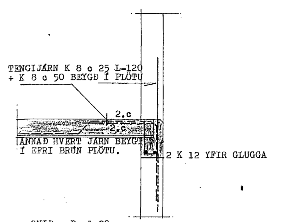
SNID - B 1:20
