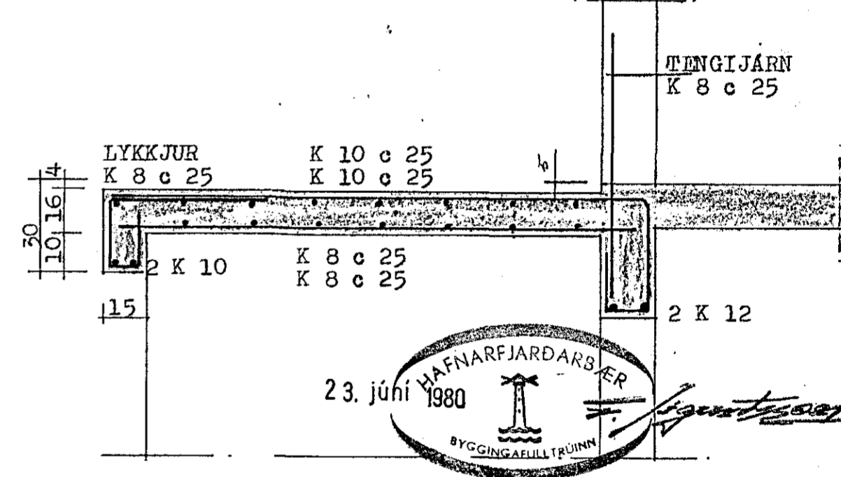
SNID - D 1:20
