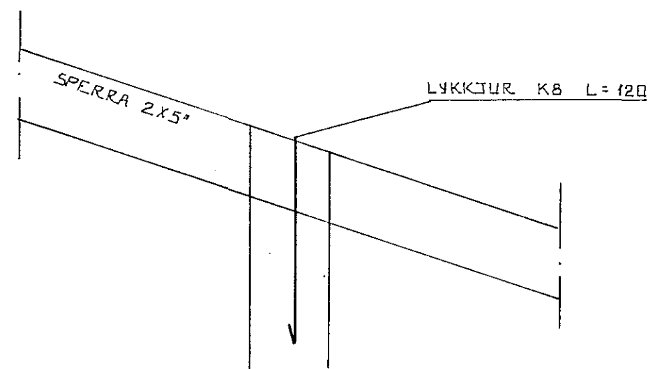
SNID D-D 1:10
