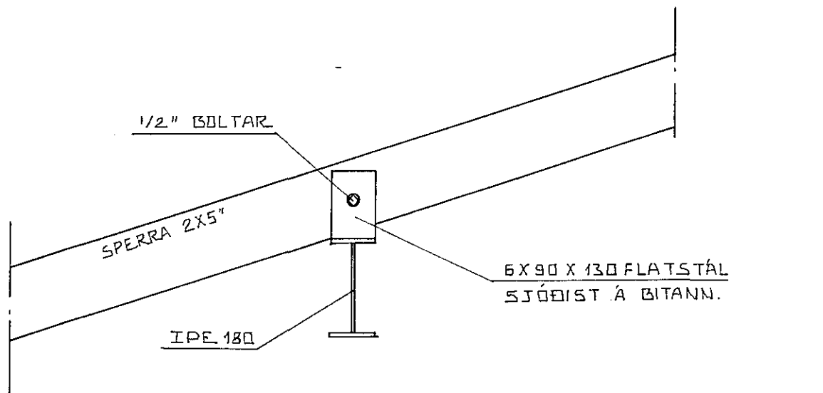
SNID B-B 1:10
