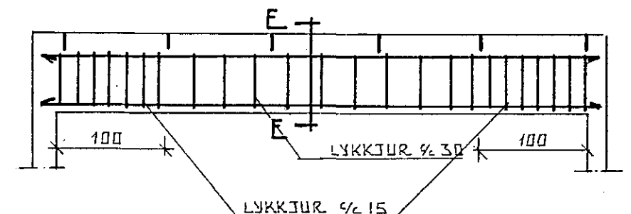
LANGSNID Í BITA 1:50
