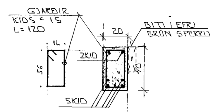
SNÍÐ 14 1:20
