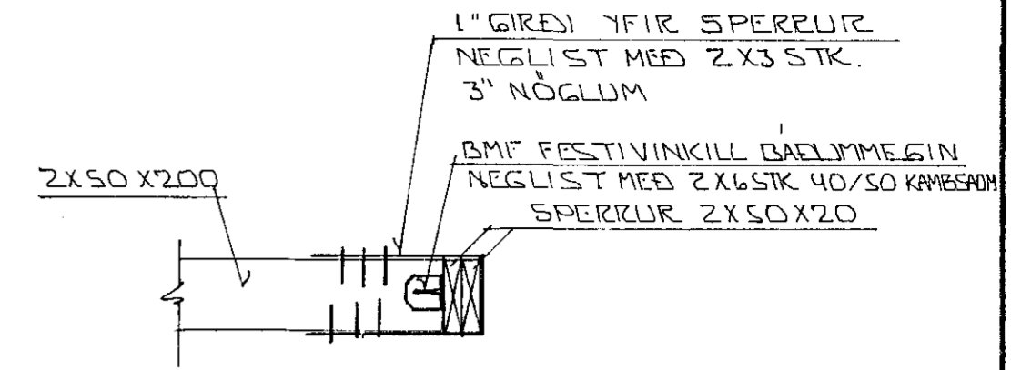
SNÍÐ 13 1:20
