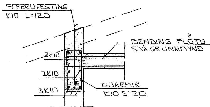
SNID A Í BITA YFIR GLUGGUM 1:20
