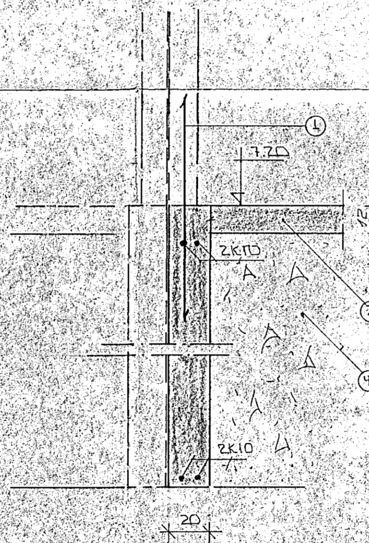
SNID 4 1:20
