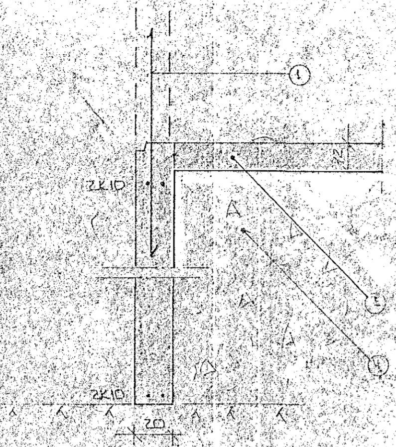
SNID 1 I UTVEGGI 1:20
