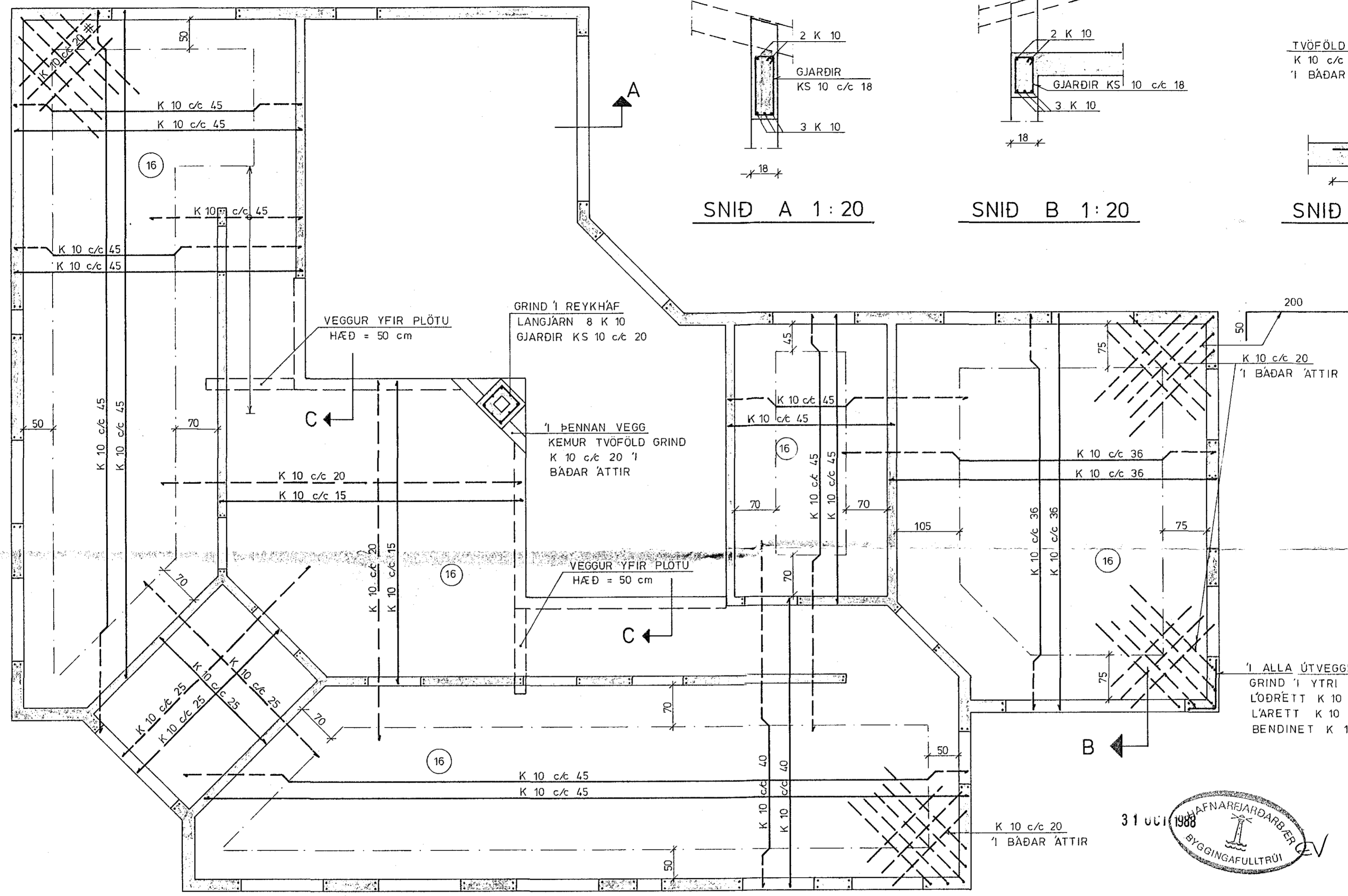
GRUNNMYND 1 : 50
