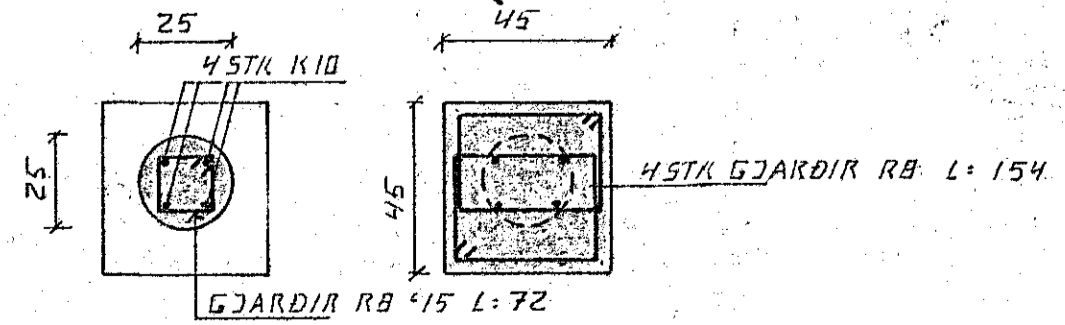
SÚLA S5. 1:20
