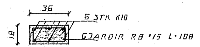
SÚLA S3. 1:20
