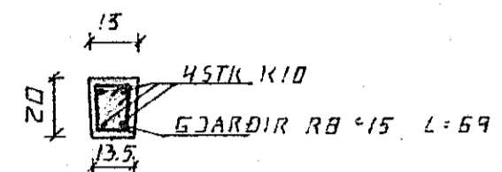
SÚLA S2. 1:20
